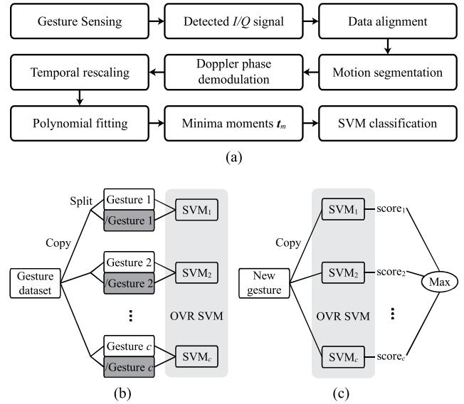
图 9. 手势识别流程图。(a) 信号处理。(b) OVR SVM 的训练。(c) 基于已训练 OVR SVM 的手势识别。
