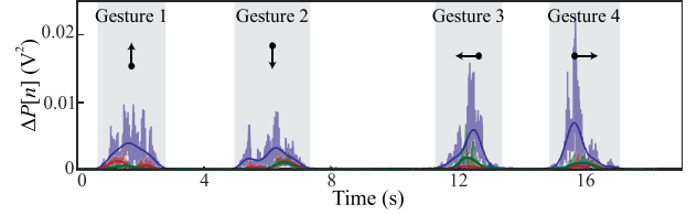
图17. 基于图16中检测到的信号的微分功率 \Delta P[n] 以及移动平均 \Delta P_{60}[n] 进行的分割过程。
