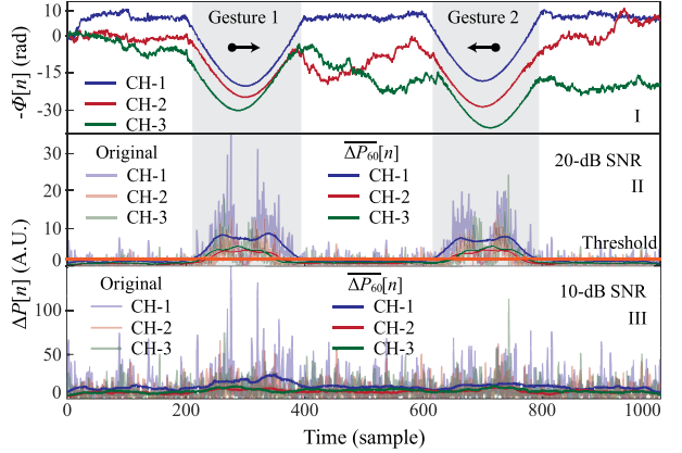
图12. 两个连续“向右”和“向左”手势的分段结果。子图I: 20 dB SNR下的解调多普勒相位。子图II: 20 dB SNR下模拟基带信号的 \Delta P[n] 和 \Delta P_{60}[n] ，以及用于分段的阈值。子图III: 10 dB SNR下模拟基带信号的 \Delta P[n] 和 \Delta P_{60}[n] 。
