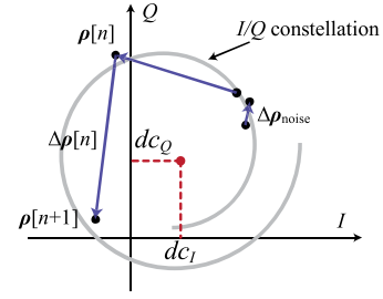
图8. \Delta \rho[n] 和 \rho_{\text{noise}} 在 I/Q 星座图中的示意图。
