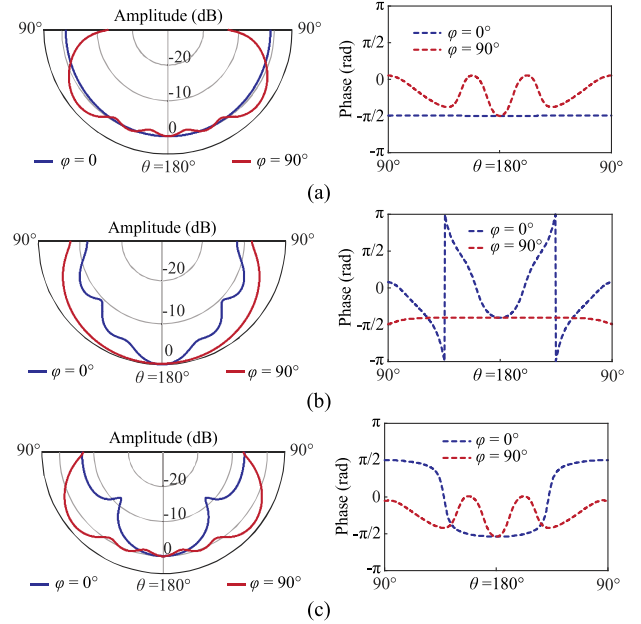
图5. 通过(6)式计算的不同孔径尺寸下的散射方向图。(a) w = 2 cm, l = 15 cm。(b) w = 15 cm, l = 2 cm。(c) w = 8 cm, l = 15 cm。
