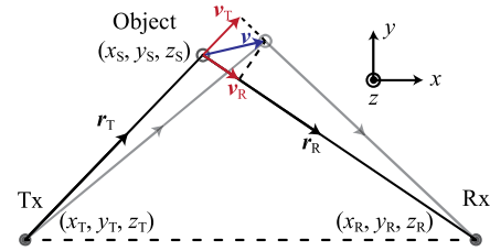
图6. 双基地DRS检测到的多普勒相位。
