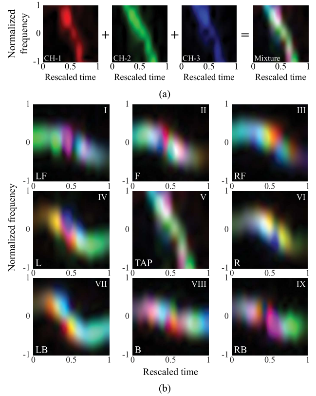
图 25. 不同手势产生的时频谱图。(a) 单色和全色谱图。(b) 用于基于 DCNN 分类的全色多普勒谱图。
