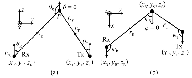
图4. 移动手掌散射分析的双基地模型。(a) yOz 视图。(b) xOy 视图。
