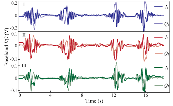
图 16. 实验 I/Q 信号来自天线 R_1 、 R_2 , 和 R_3 , 分别检测到的连续四次“向前”、“向后”、“向左”和“向右”手势。
