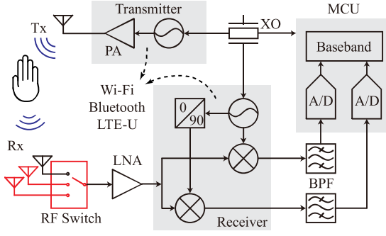
图 1. 通过重构 Wi-Fi 和 LTE-U 信道实现 TDM-SIMO DRS。红色绘制的设备为新增设备。
