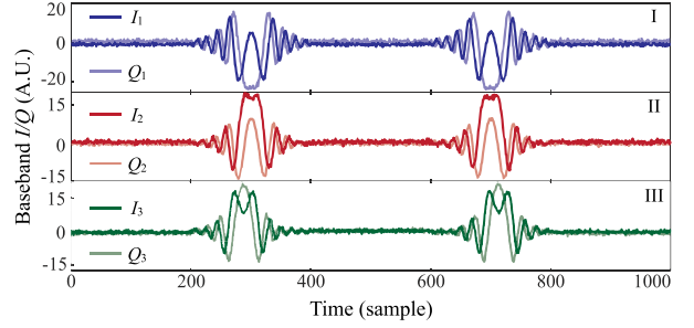
图11. 由 R_1 , R_2 , 和 R_3 天线分别“检测”到的两个连续“向右”和“向左”手势所产生的模拟 I/Q 信号。
