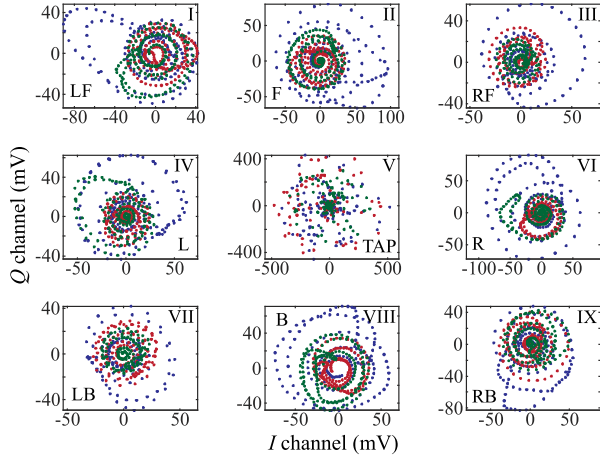
图19. 实验中执行手势的星座图。
