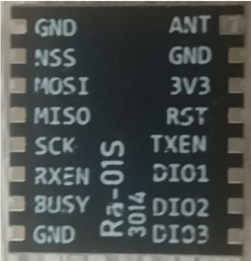
图 2 Ra-01S 管脚图
