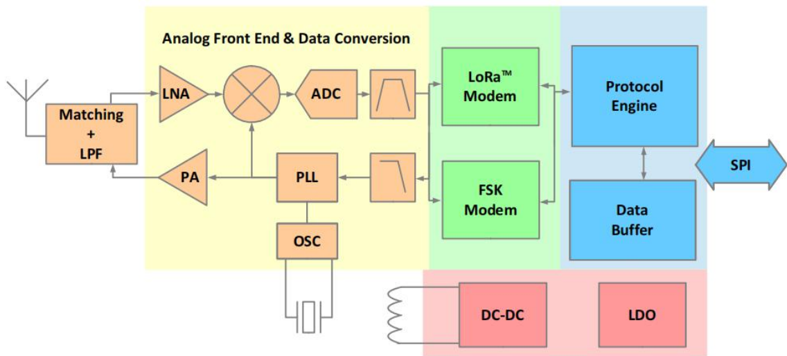
图 1 SX1268 功能方框图
