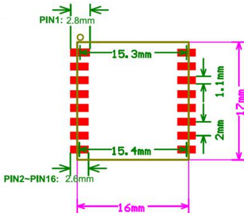
图 6 Ra-01S 模块 PCB 封装图
