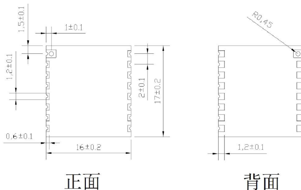
图 4 Ra-01S 模块尺寸平面图
