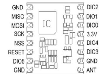
2) Pin Out
