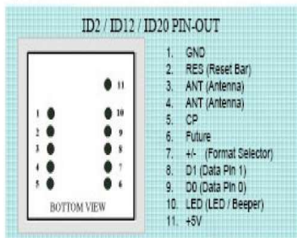
2) Pin Out
