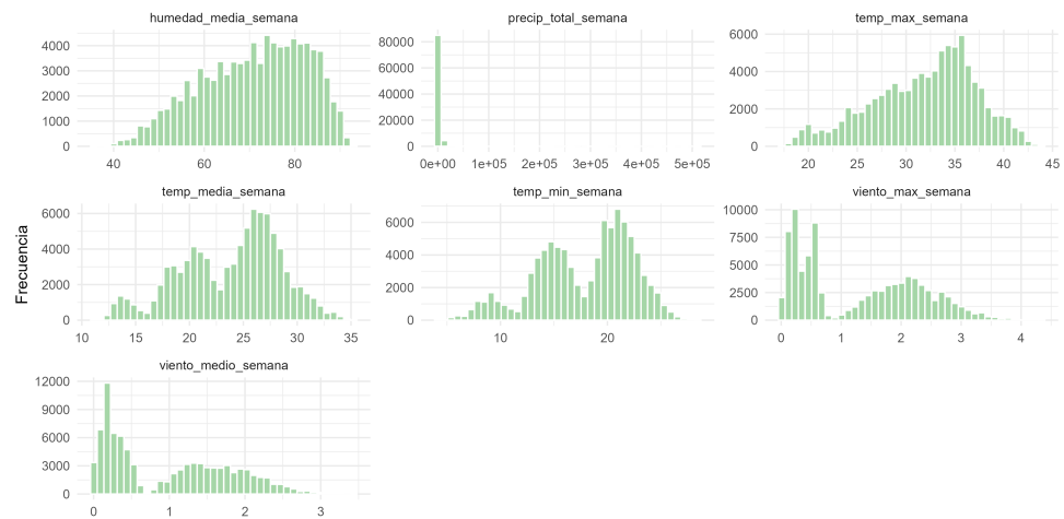
Figura 5.10: Histogramas de las variables climáticas semanales en la tabla agrupada ( N_{\text{agr}} = 90,128 ).
