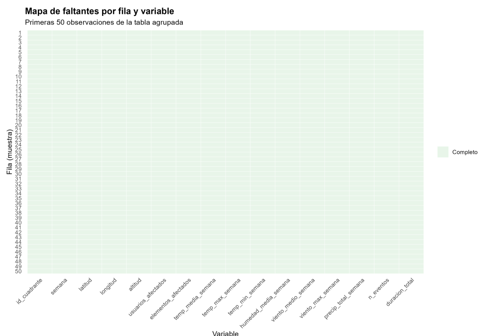
Figura 5.4: Mapa de faltantes por fila y variable en la tabla agrupada cuadrante \times semana ( N_{\text{agr}} = 90,128 ; muestra de 50 filas).
