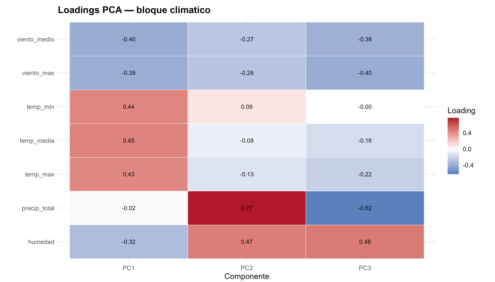
Figura 5.43: Loadings de las tres primeras componentes principales del bloque climático.
