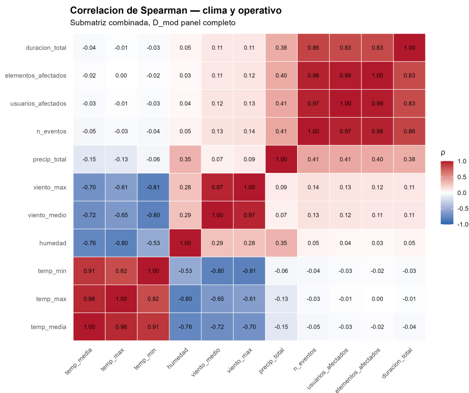
Figura 5.36: Mapa de calor de correlaciones de Spearman entre variables climáticas y operativas en D_{mod} .
