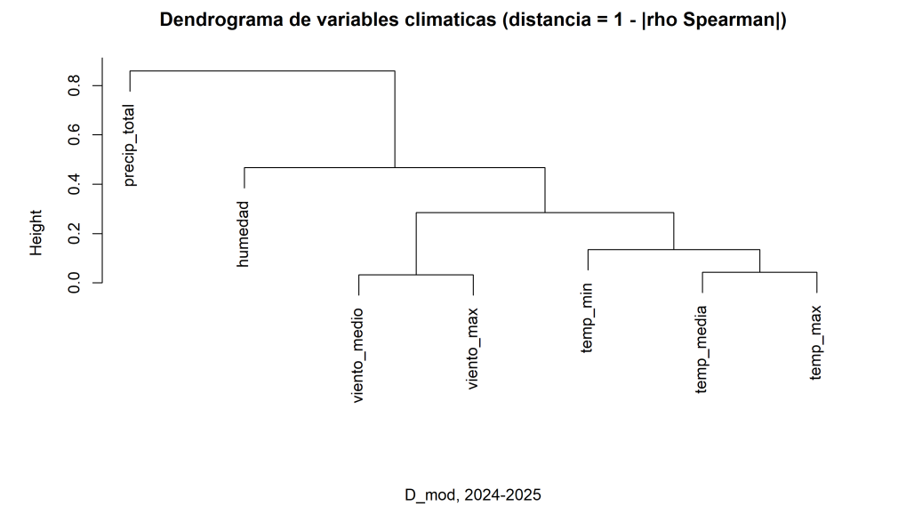
Figura 5.44: Dendrograma de variables climáticas (distancia = 1 - |\rho_{\text{Spearman}}| ).
