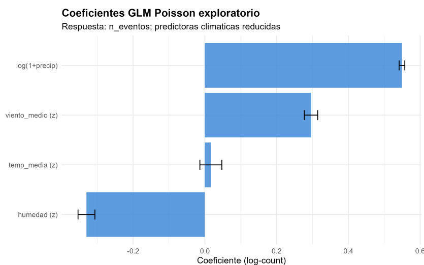
Figura 5.44: Coeficientes del GLM Poisson exploratorio n\_eventos \sim clima reducido (diagnóstico EDA).
