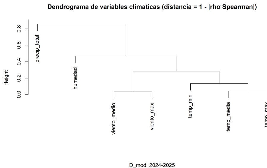
Figura 5.43: Dendrograma de variables climáticas (distancia basada en correlación de Spearman; Sección 3.1.2).
