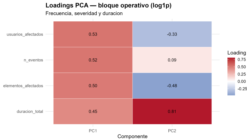
Figura 5.45: Loadings PCA del bloque operativo en escala logarítmica desplazada. depuración cuantitativa y la construcción de matrices de diseño de la Etapa 4.
