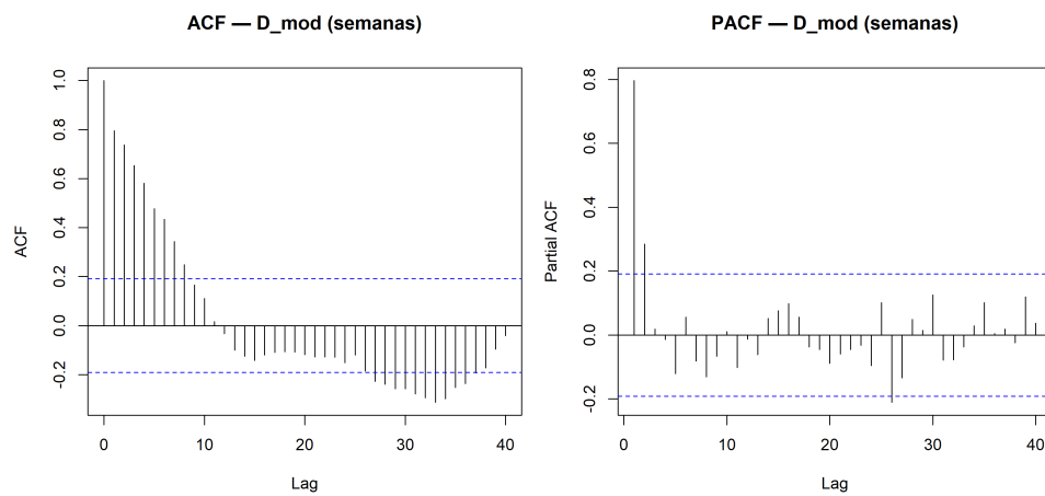
Figura 5.29: ACF y PACF de la serie semanal de eventos en D_{\text{mod}} .
