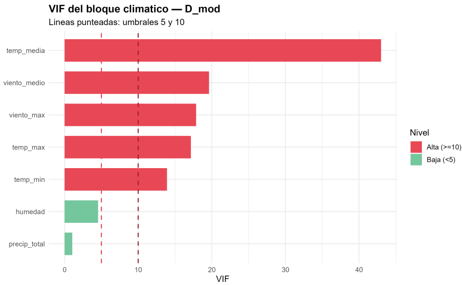
Figura 5.40: VIF del bloque climático en modelo auxiliar n\_eventos \sim clima (D_{mod}) .
