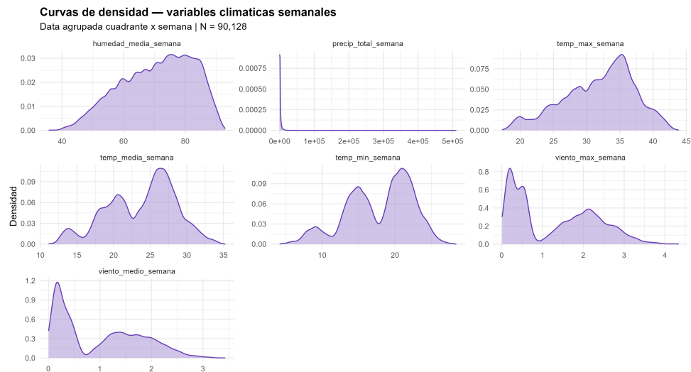
Figura 5.14: Curvas de densidad de las variables climáticas semanales ( N_{agr} = 90.128 ).
