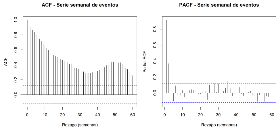
Figura 5.24: ACF y PACF de la serie semanal de eventos (rezagos en semanas).
