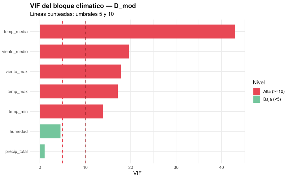
Figura 5.40: VIF del bloque climático en modelo auxiliar n_eventos \sim clima ( D_{\text{mod}} ).
