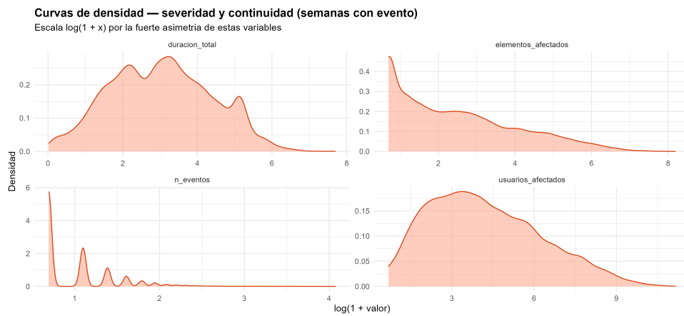
Figura 5.17: Curvas de densidad de severidad y continuidad en escala \log(1+x) (semanas con evento).
