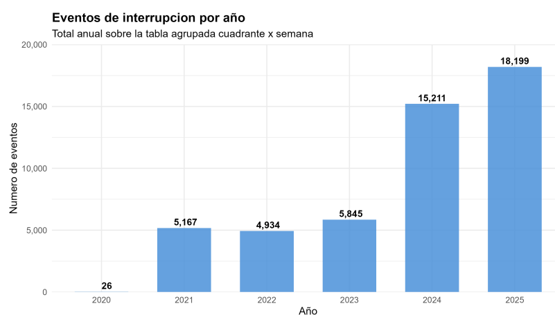
Figura 5.21: Total anual de eventos de interrupción sobre la tabla agrupada.
