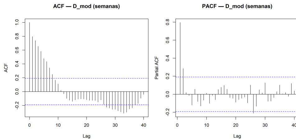
Figura 5.29: ACF y PACF de la serie semanal de eventos en D_{mod} .
