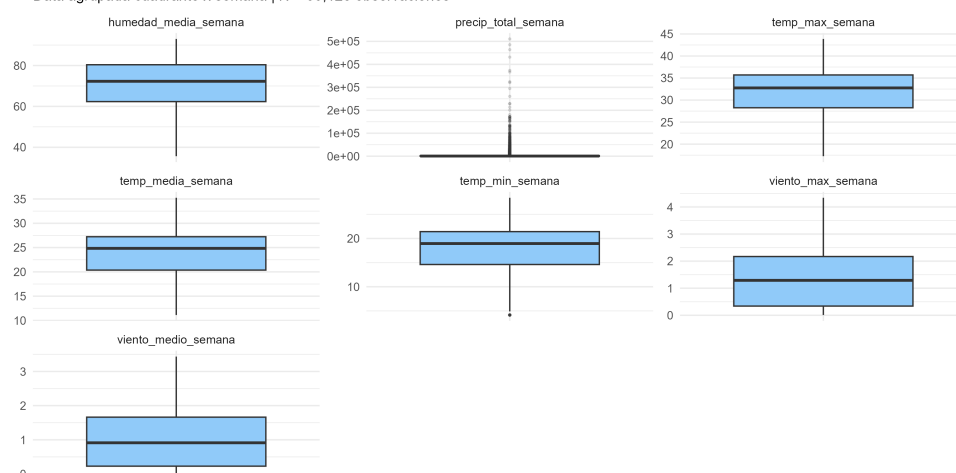
Figura 5.8: Diagramas de caja de las variables climáticas semanales en la tabla agrupada ( N_{\text{agr}} = 90.128 ).
