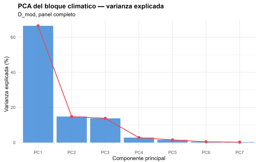
Figura 5.41: Varianza explicada por componentes principales del bloque climático.
