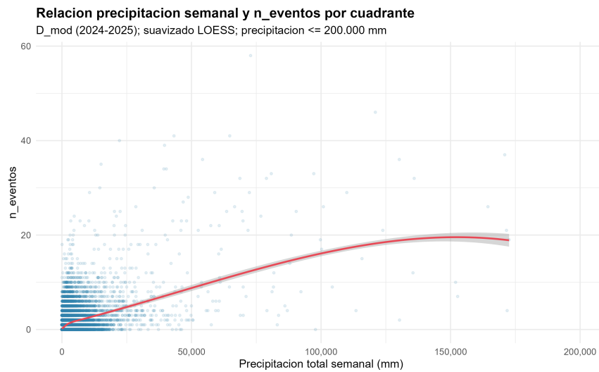
Figura 5.33: Dispersión entre precipitación semanal y n_{eventos} por cuadrante en D_{mod} .
