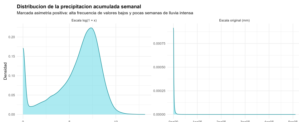
Figura 5.18: Distribución de la precipitación acumulada semanal en escala original y \log(1 + x) ( N_{agr} = 90.128 ).
