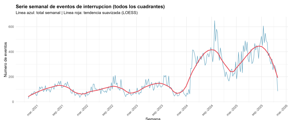
Figura 5.20: Serie semanal de eventos de interrupción (suma sobre los cuadrantes) con tendencia LOESS, 2021–2025.
