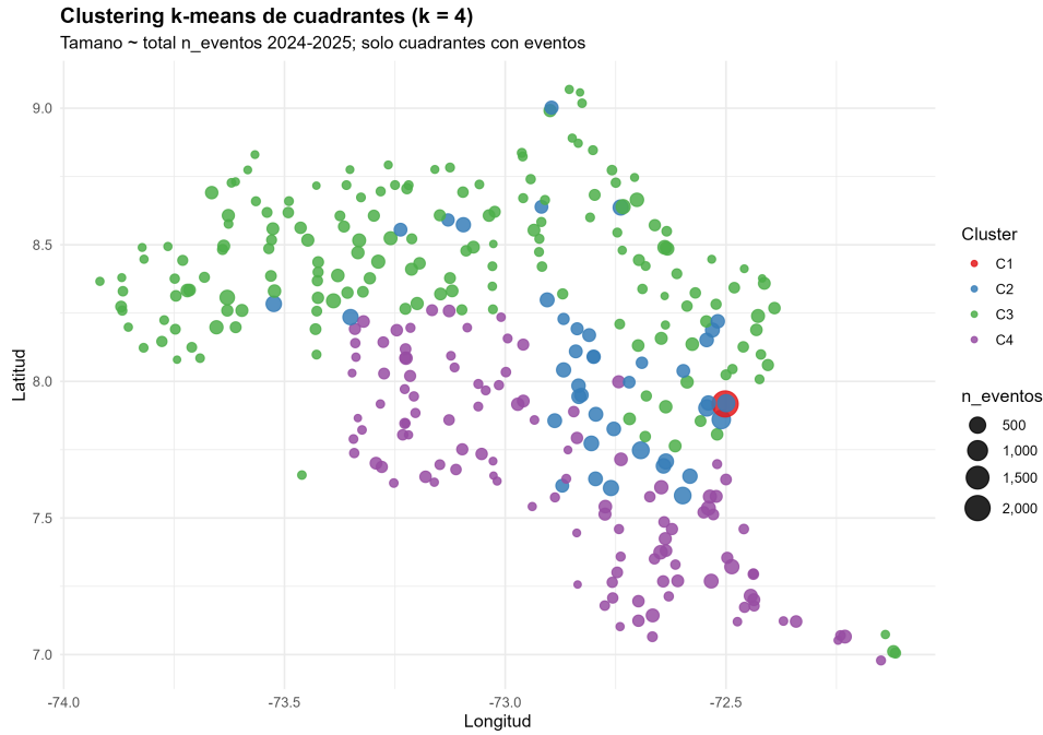
Figura 5.50: Clustering k-means de cuadrantes ( k = 4 ) en D_{\text{mod}} .
