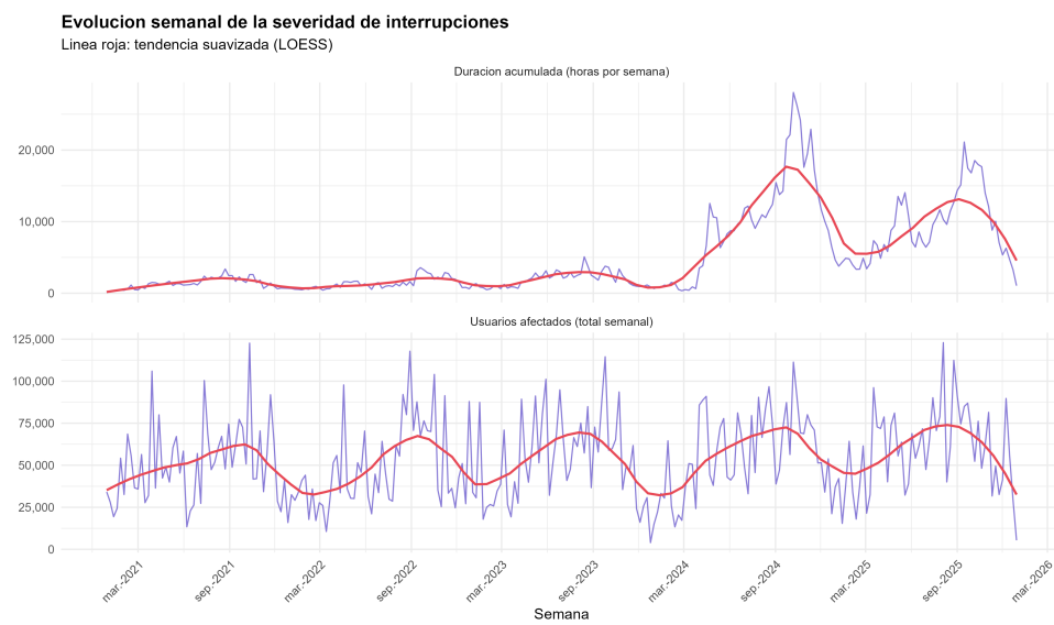
Figura 5.25: Evolución semanal de usuarios afectados y duración acumulada, con tendencia LOESS.
