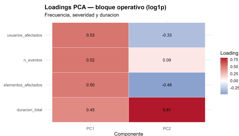
Figura 5.45: Loadings PCA del bloque operativo en escala \log(1+x) .
