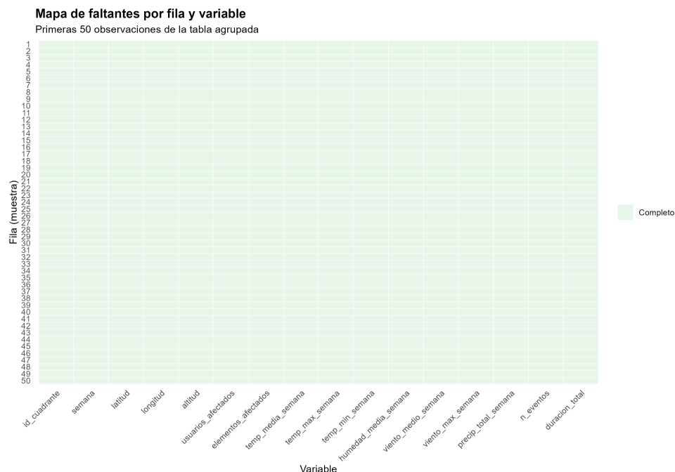
Figura 5.3: Mapa de faltantes por fila y variable en la tabla agrupada cuadrante \times semana ( N_{\text{agr}} = 90.128 ; muestra de 50 filas).
