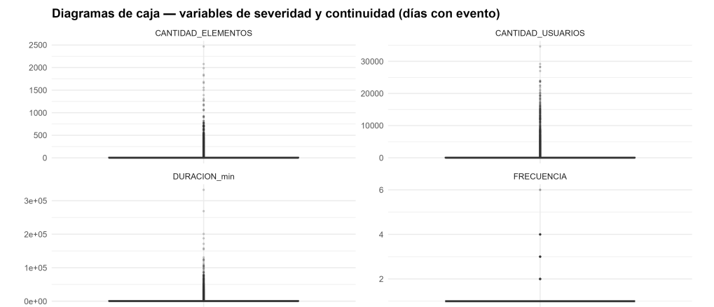
Figura 5.6: Diagramas de caja de las variables de severidad y continuidad en días con evento.
