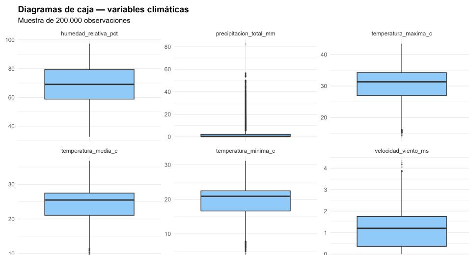
Figura 5.4: Diagramas de caja de las variables climáticas (muestra de 200.000 observaciones).
