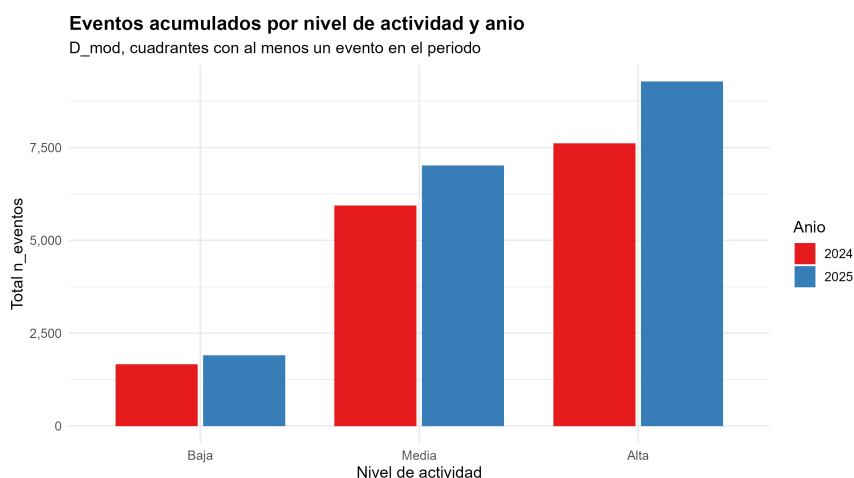
Figura 5.48: Eventos acumulados por nivel de actividad y año en D_{mod} .
