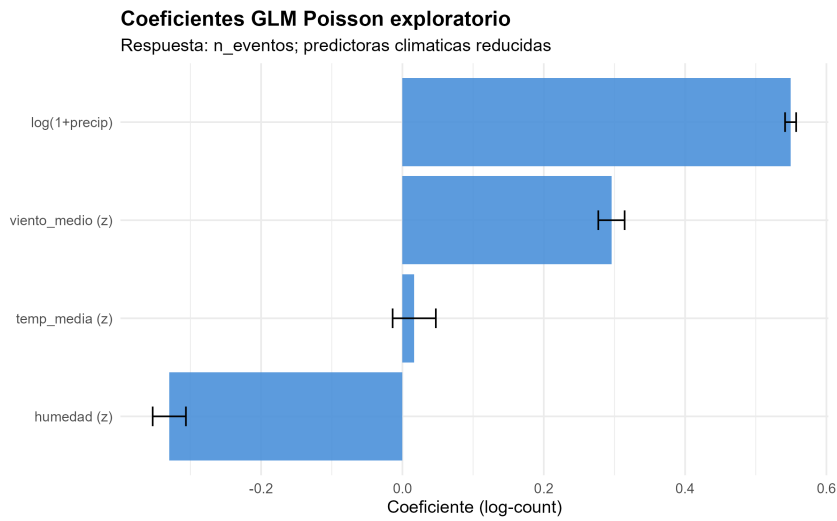
Figura 5.44: Coeficientes del GLM Poisson exploratorio n\_eventos \sim \text{clima reducido} (diagnóstico EDA).
