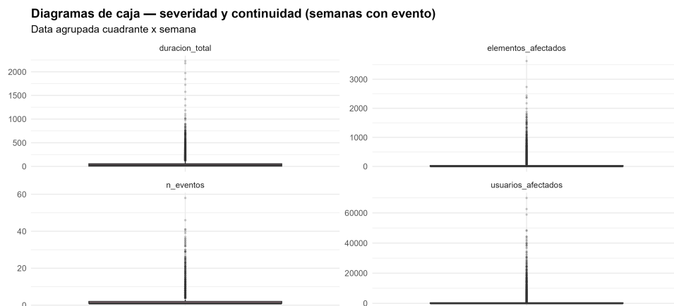
Figura 5.10: Diagramas de caja de severidad y continuidad en semanas con evento (tabla agrupada).
