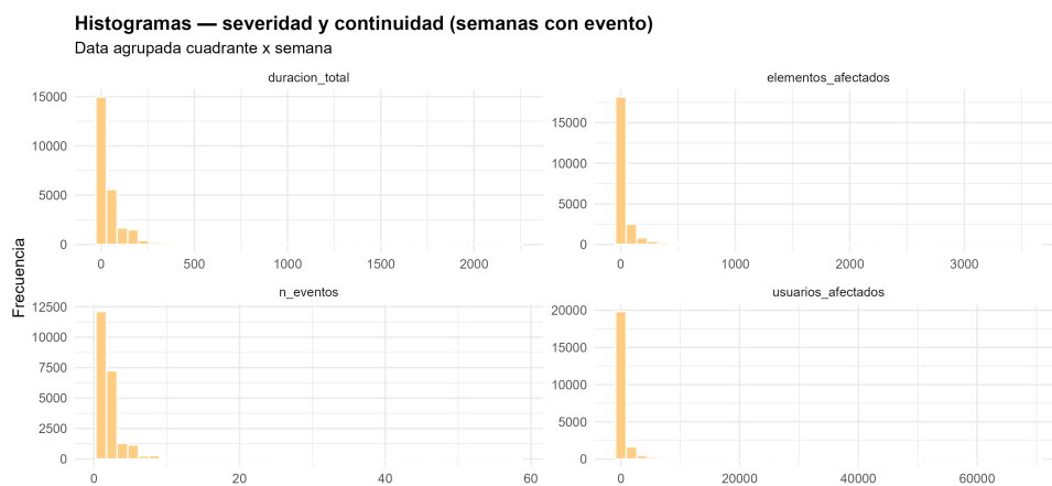
Figura 5.11: Histogramas de severidad y continuidad en semanas con evento (tabla agrupada).
