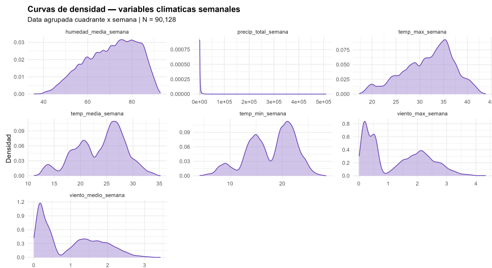
Figura 5.14: Curvas de densidad de las variables climáticas semanales ( N_{\text{agr}} = 90.128 ).
