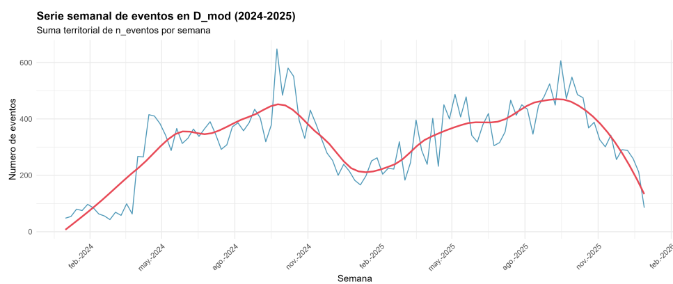
Figura 5.27: Serie semanal de eventos sobre D_{\text{mod}} (2024–2025) con tendencia LOESS.
