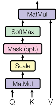
縮放點積注意力
