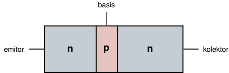
Skema (digambar ulang) — penampang transistor sambungan n-p-n
