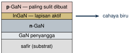
Skema (digambar ulang) — susunan lapisan LED biru berbasis GaN
