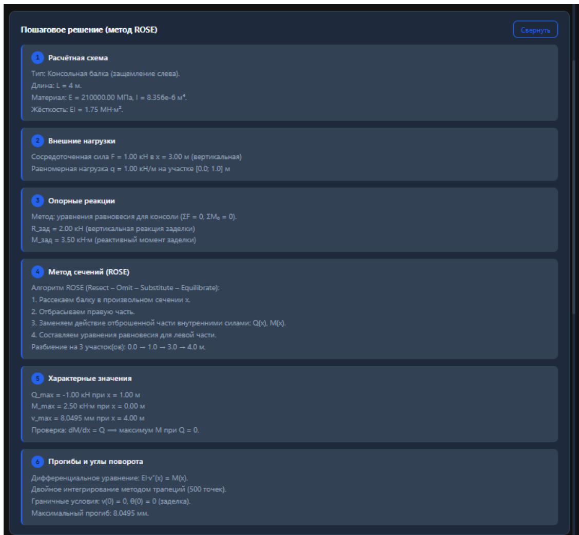
Рис. 1.11. Виджет пошагового решения задачи
