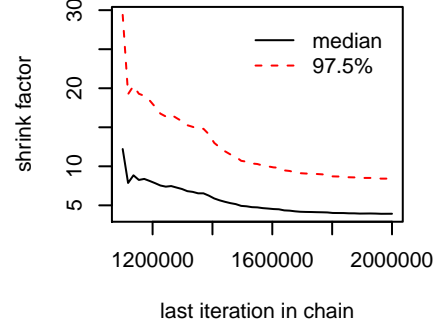
posterior
