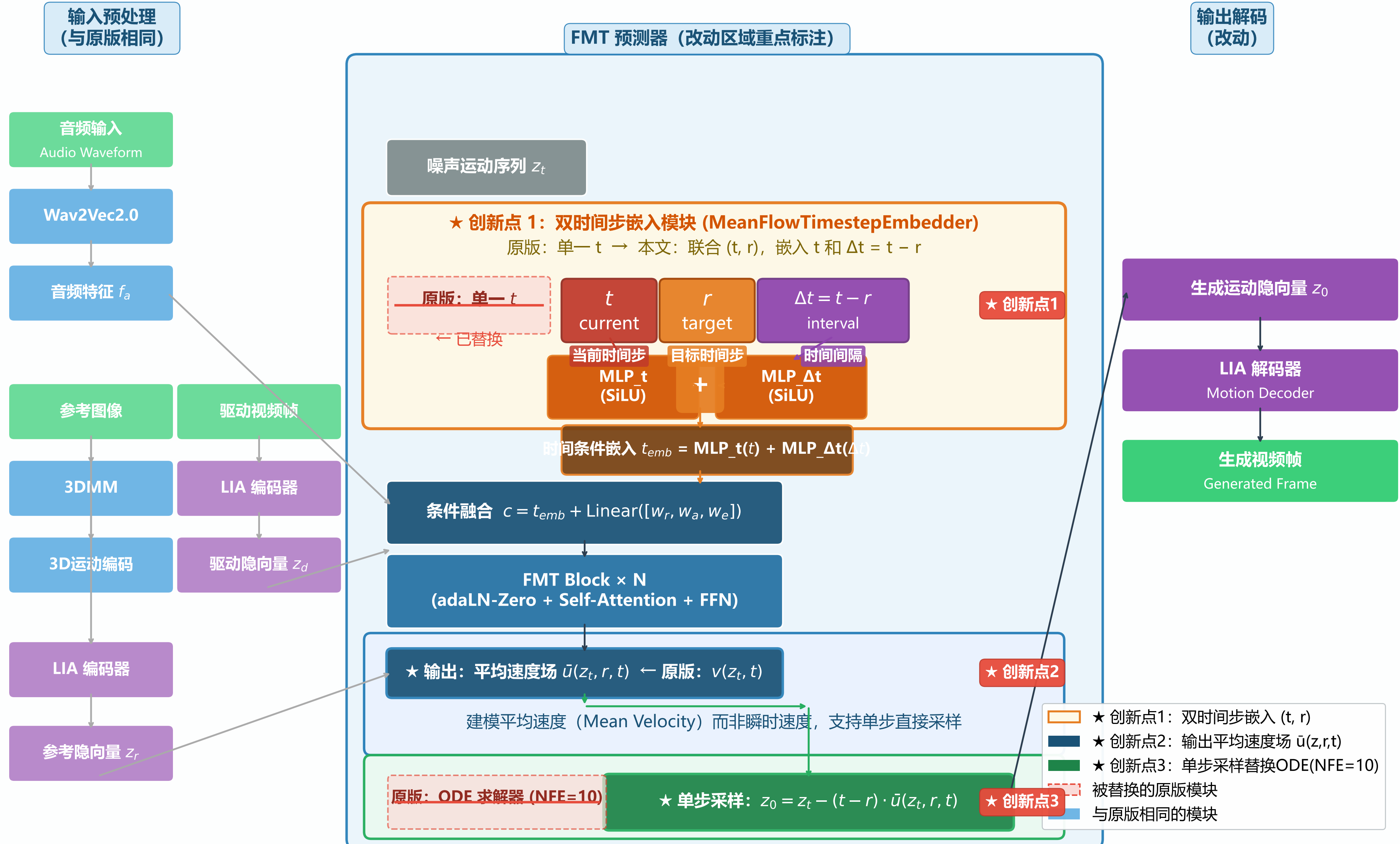
图 3-2: MF-FLOAT 相对于原始 FLOAT 的改动标注图。红色虚线框为被替换模块, 橙色实线框为创新点, 绿色为新增单步采样。
