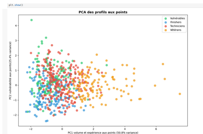
Figure 21: Annexe 21 : PCA – clustering soumissions sur espace points.
