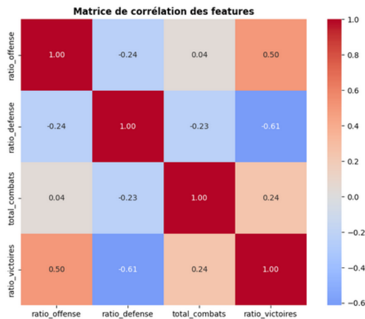
Figure 3: Annexe 3 : Matrice de corrélation des features principales.
