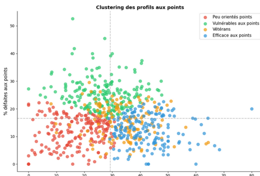
Figure 13: Annexe 13 : Clustering des profils aux points ( K = 4 ).
