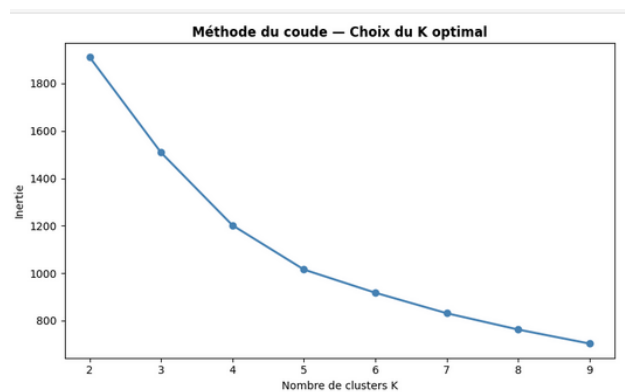
Figure 5: Annexe 5 : Méthode du coude – choix du K optimal.
