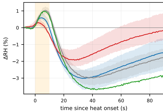
(d) Coupled humidity response
