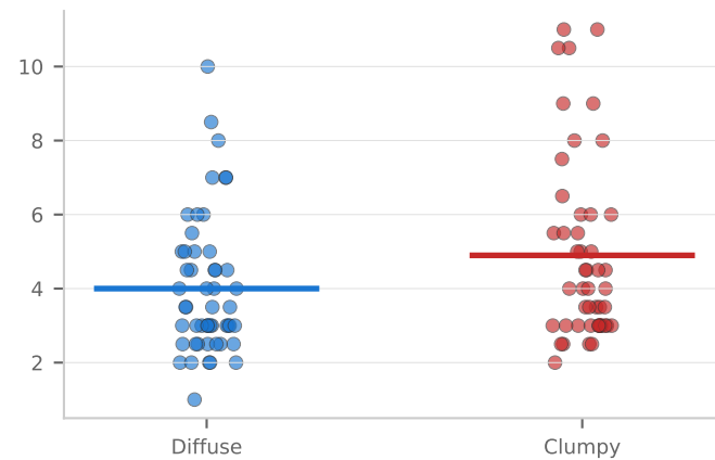
seq_typing_max_run d=-0.41 p=0.043
