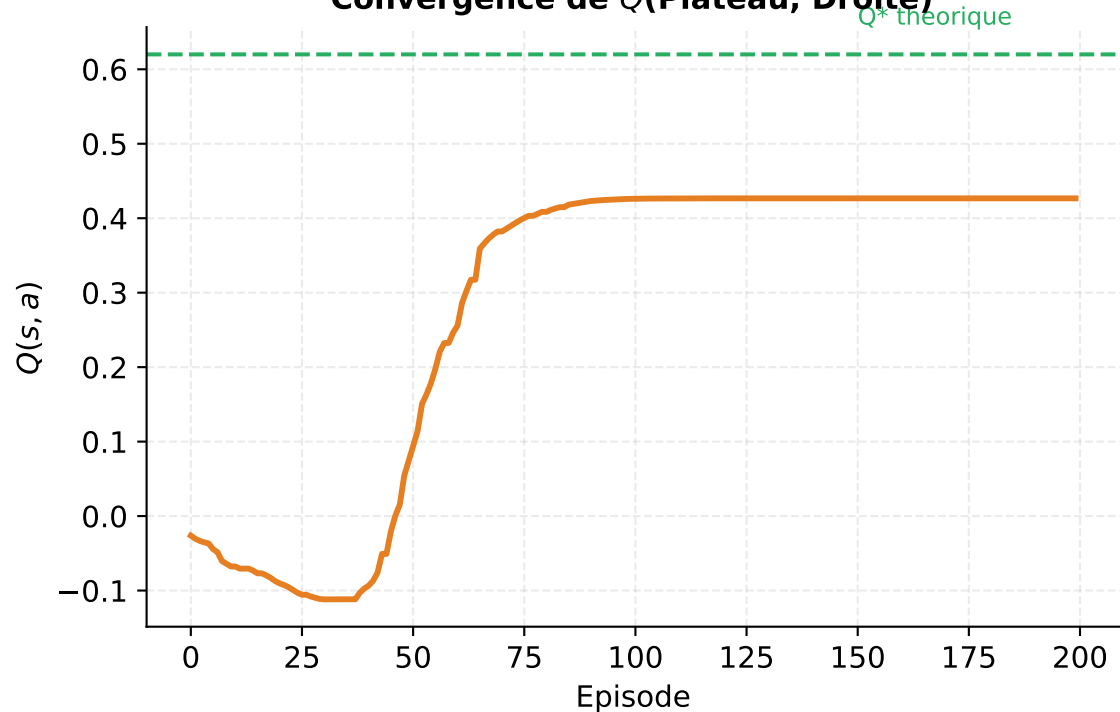
Convergence de Q (Plateau, Droite)
