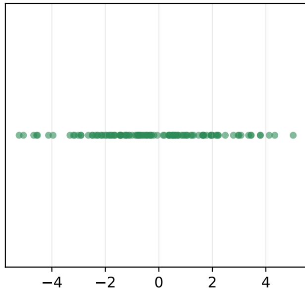
Projection sur PC1 : réduit à 1 dimension
