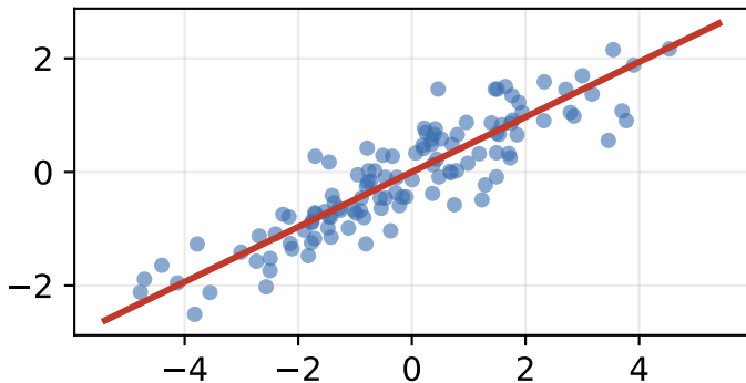
Données 2D + axe principal PC1
