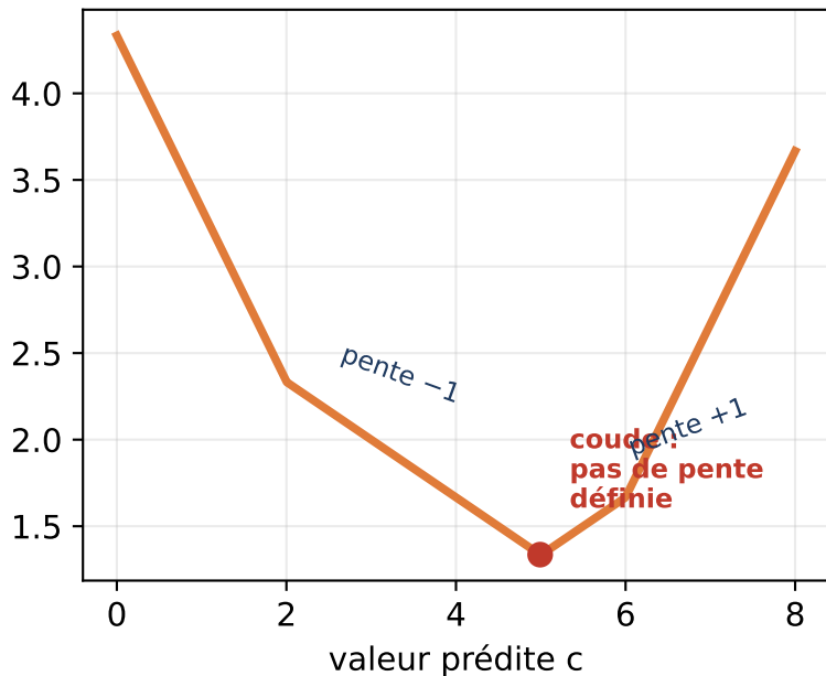
MAE : des coudes (non lisse)
