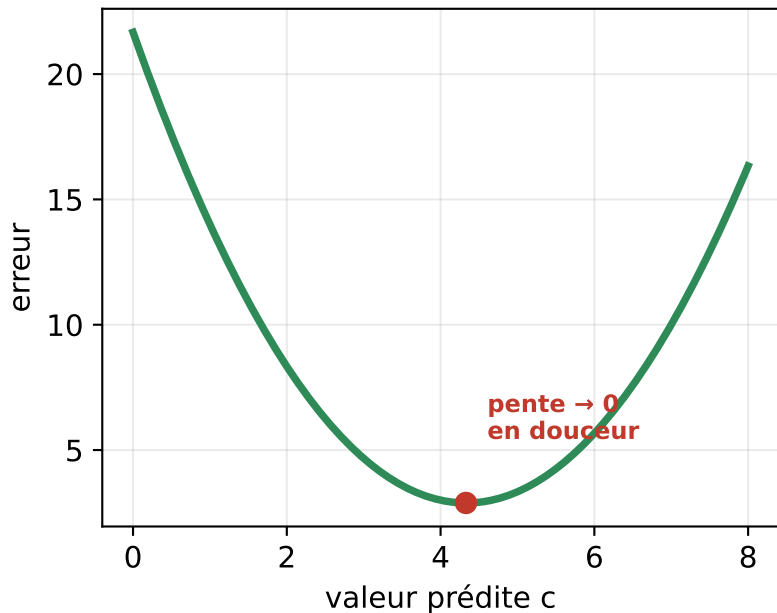
MSE : une cuvette lisse
