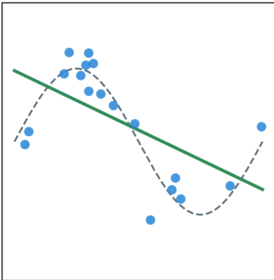
degré 1 — trop simple (sous-ajustement)
