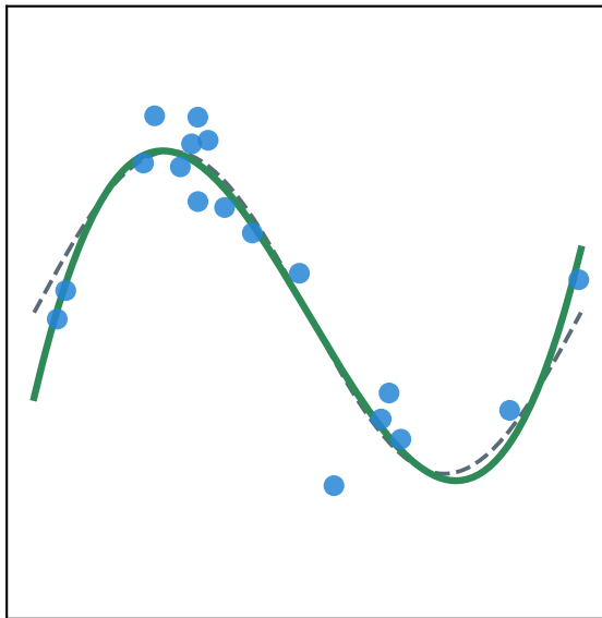
Mêmes données, trois degrés (pointillé = vraie fonction) degré 3 — bon dosage
