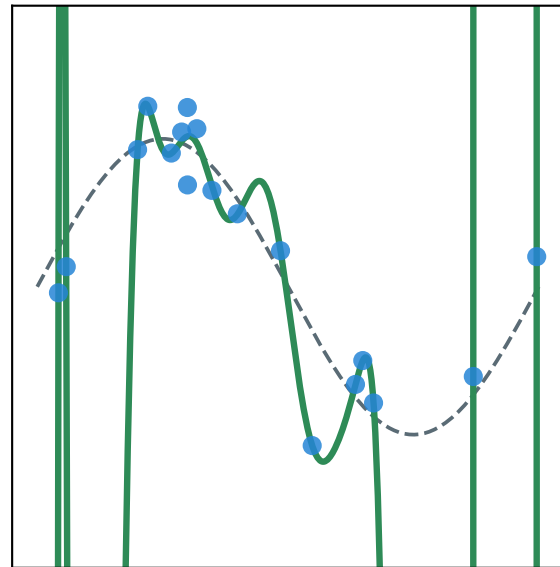
degré 15 — trop complexe (sur-ajustement)
