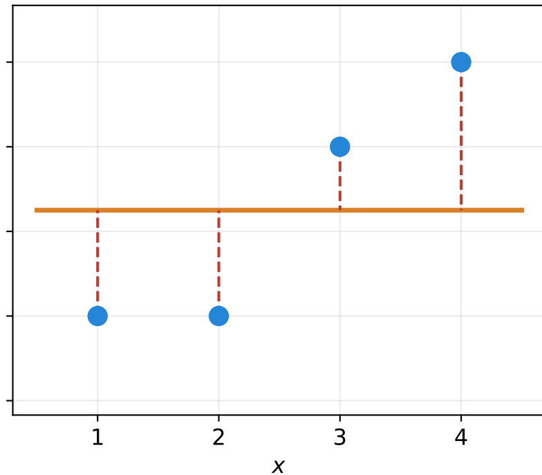
droite plate (moyenne) — MSE = 1,688
