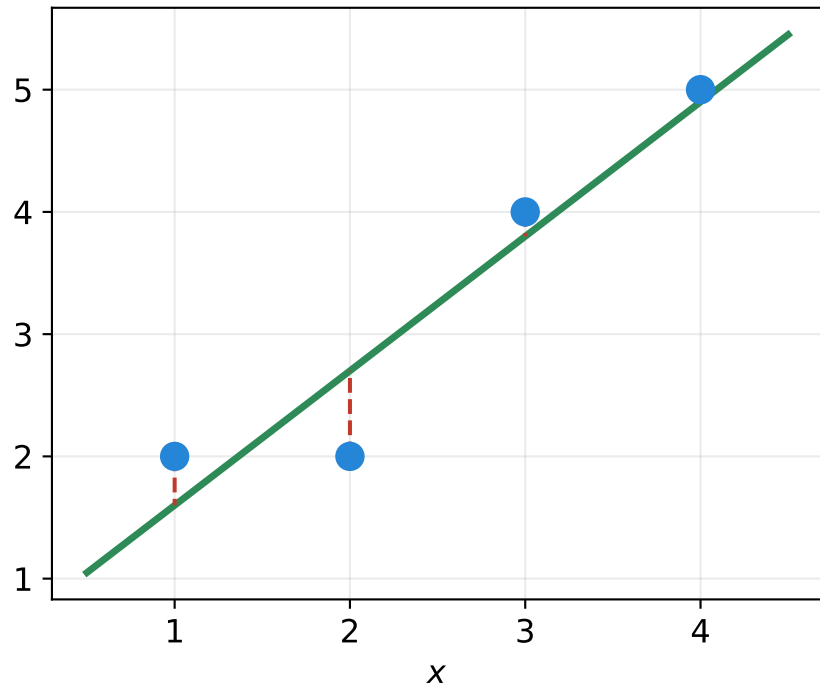
droite ajustée — MSE = 0,175
