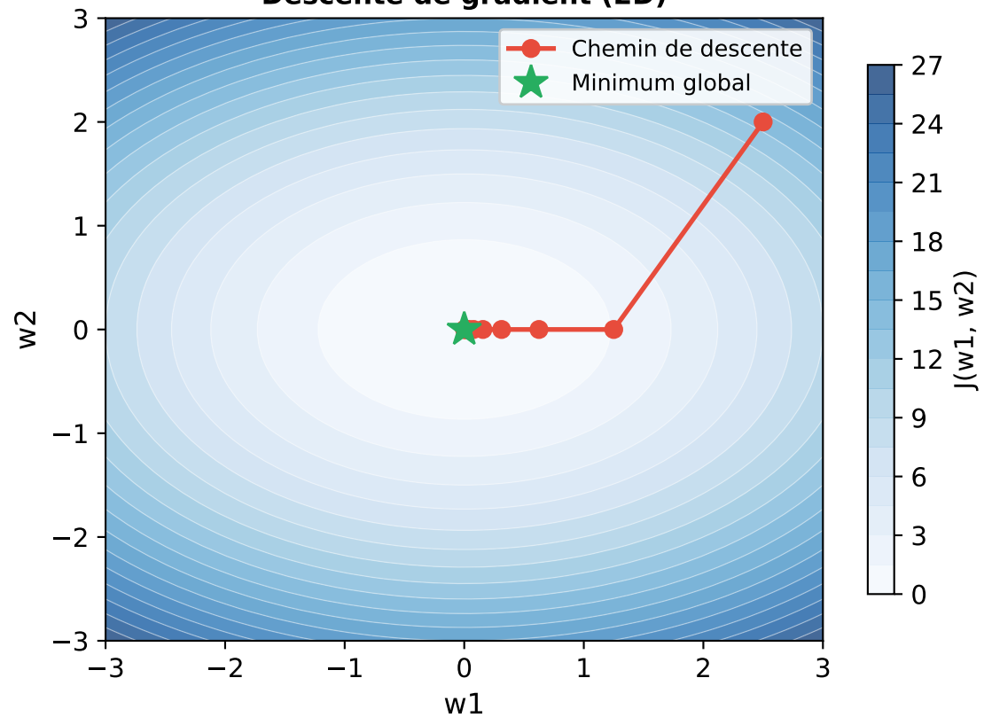
Descente de gradient (2D)
