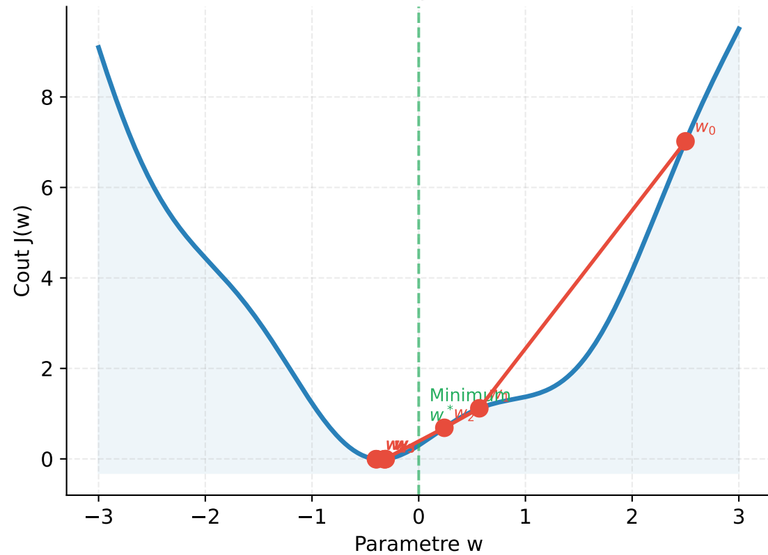
Descente de gradient (1D)
