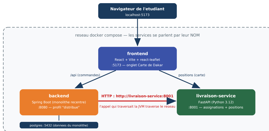
FIGURE 2 — L’orchestre : le nom du service est son adresse sur le réseau compose.
