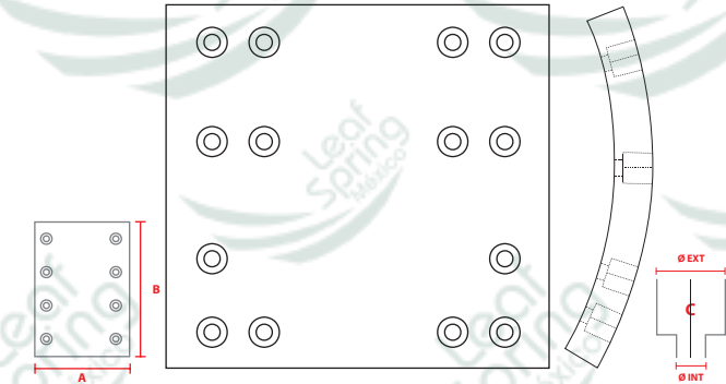
NO. PARTE FMSI / VWV1723F300
