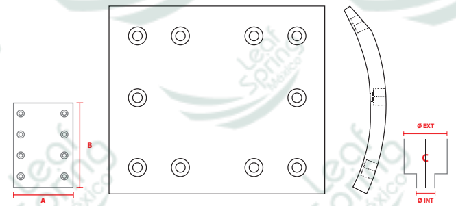
NO. PARTE FMSI HIN500R
