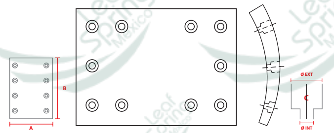
NO. PARTE FMSI 4692
