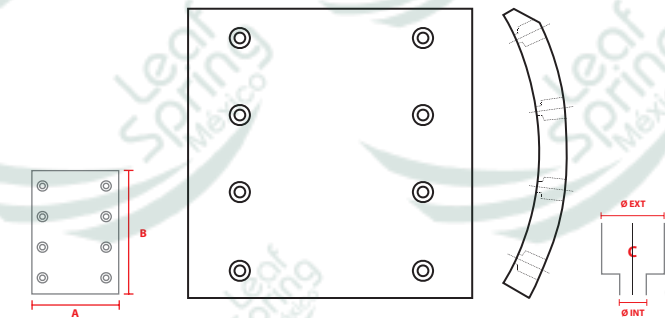
NO. PARTE FMSI 4595
