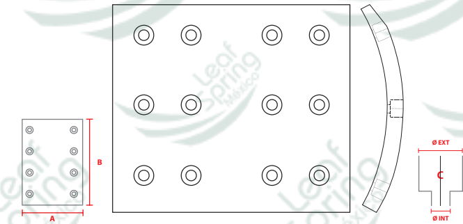
NO. PARTE FMSI IFW800R
