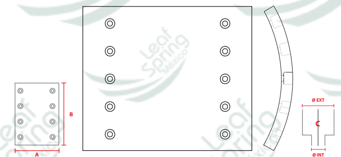
NO. PARTE FMSI BPW200
