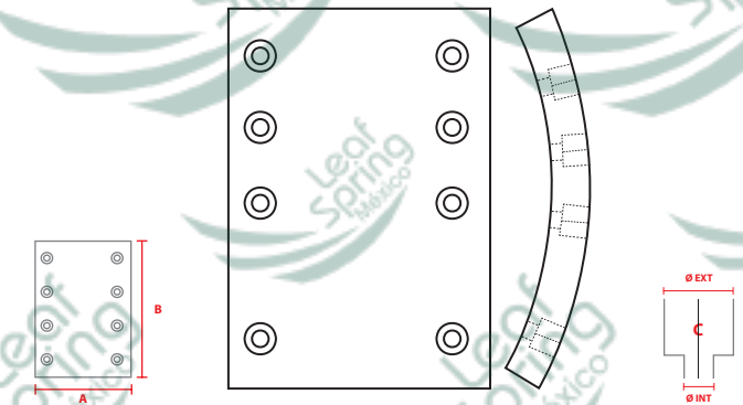
NO. PARTE FMSI 4075
