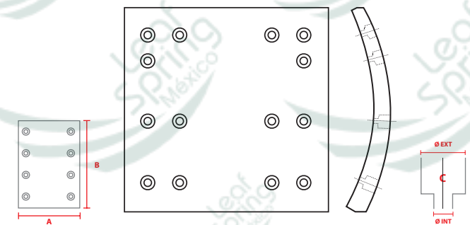
NO. PARTE FMSI 4705
