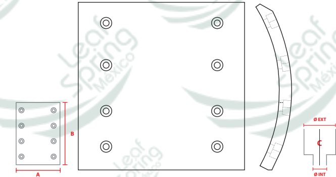
NO. PARTE FMSI / FAGTL2535R
