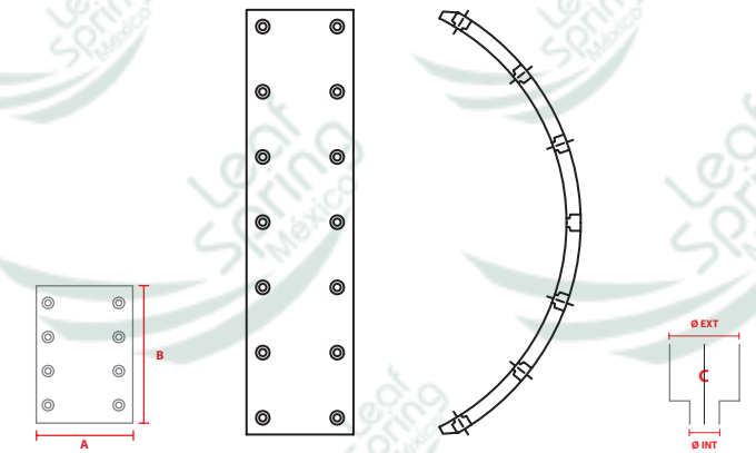
NO. PARTE FMSI 1308
