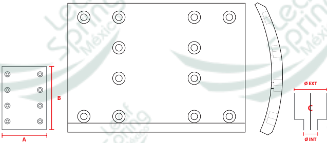
NO. PARTE FMSI C7H 540
