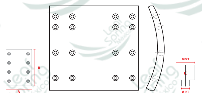
NO. PARTE FMSI 4644
