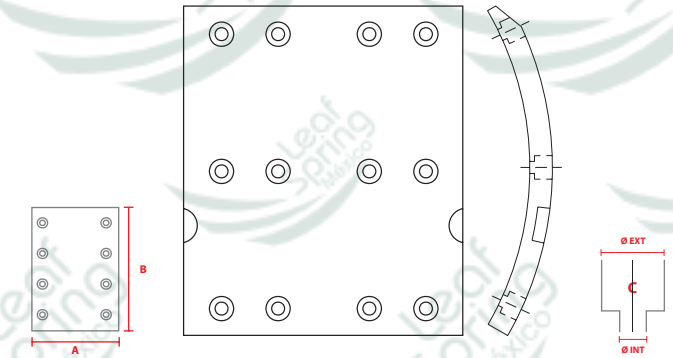
NO. PARTE FMSI 4733
