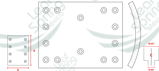
NO. PARTE FMSI STC7HR
