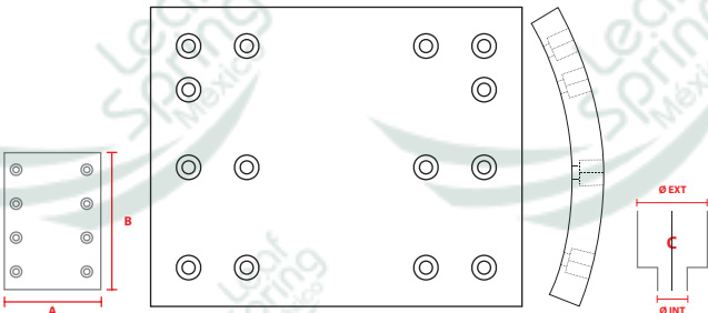
NO. PARTE FMSI / VWW1723R300
