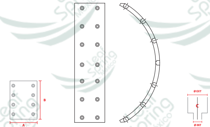
NO. PARTE FMSI 1443
