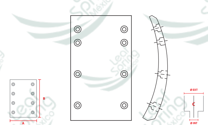
NO. PARTE FMSI 4702
