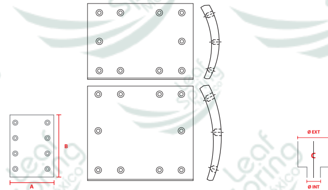
NO. PARTE FMSI / 196045500
