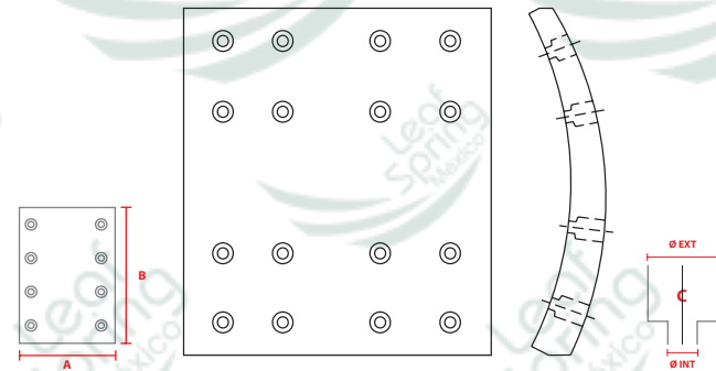
NO. PARTE FMSI 4726
