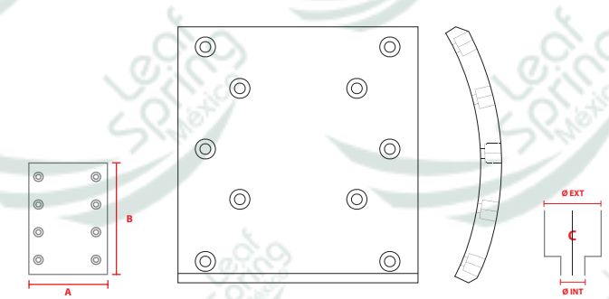
NO. PARTE FMSI / FS12F
