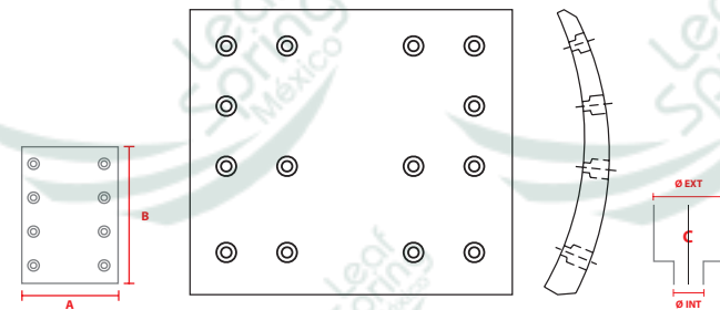
NO. PARTE FMSI 4711
