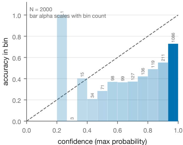
Jev (ECE = 0.281)
