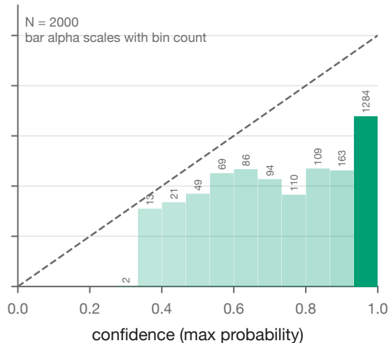
Laya (ECE = 0.307)
