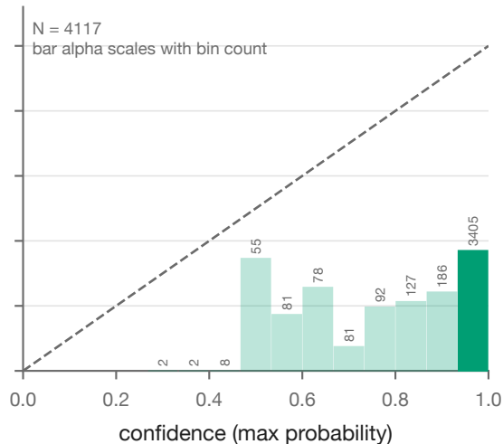
Laya (ECE = 0.610)
