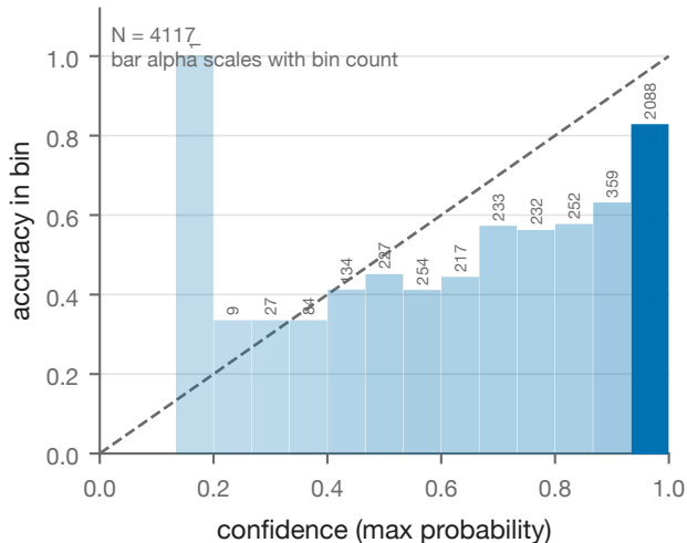
Jev (ECE = 0.166)
