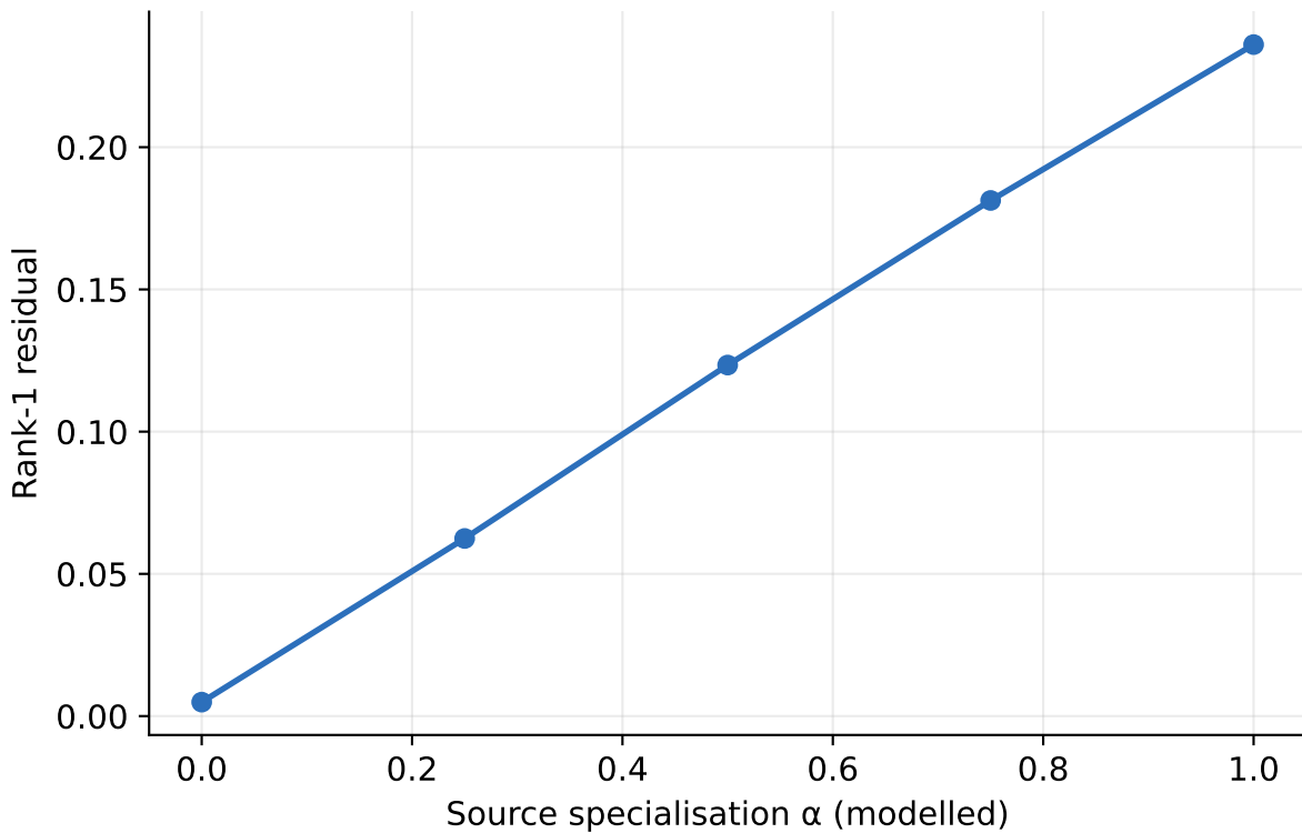
Rank-1 residual vs \alpha (OLMoE-1B-7B)
