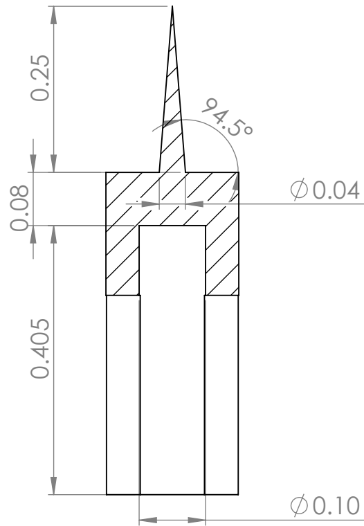
SECTION A-A SCALE 5 : 1
