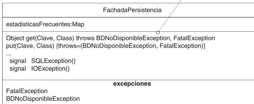
Figura 33.9. Excepciones capturadas y lanzadas por una clase.
