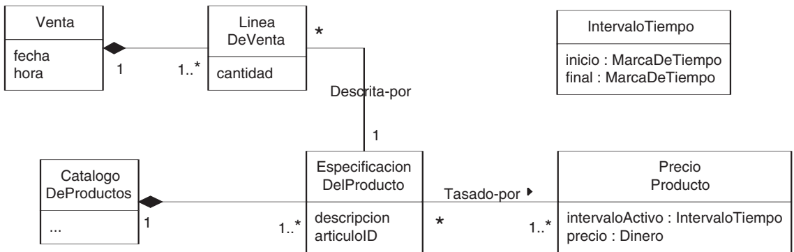
Figura 27.9. PrecioProducto e intervalos de tiempo.
