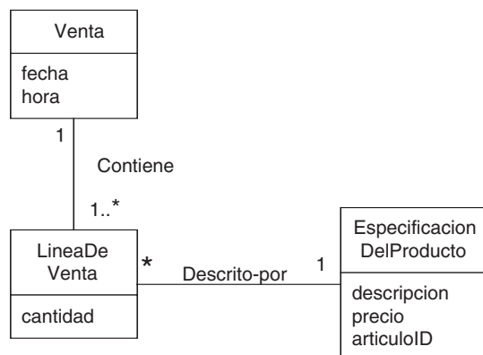
Figura 16.7. Modelo del Dominio Parcial.
