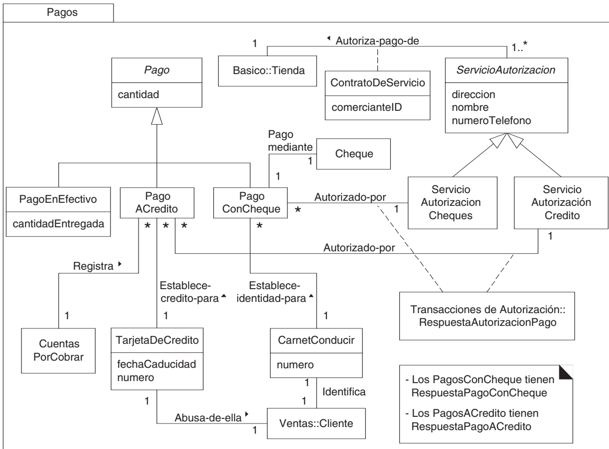
Figura 27.23. Paquete de pagos.
