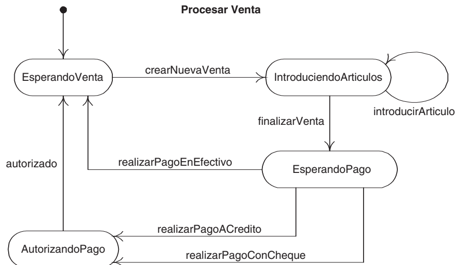
Figura 29.3. Un diagrama de estados de muestra.
