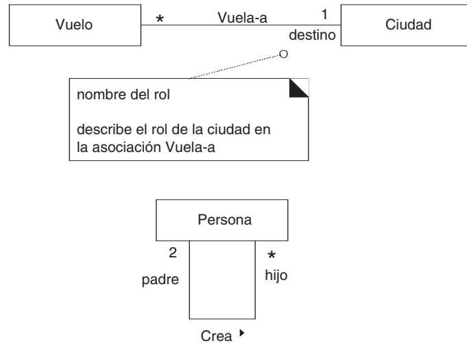
Figura 27.10. Nombres de roles.
