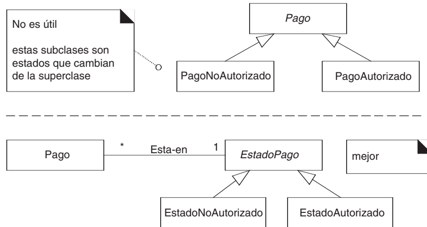
Figura 26.13. Modelado de los cambios de estado.
