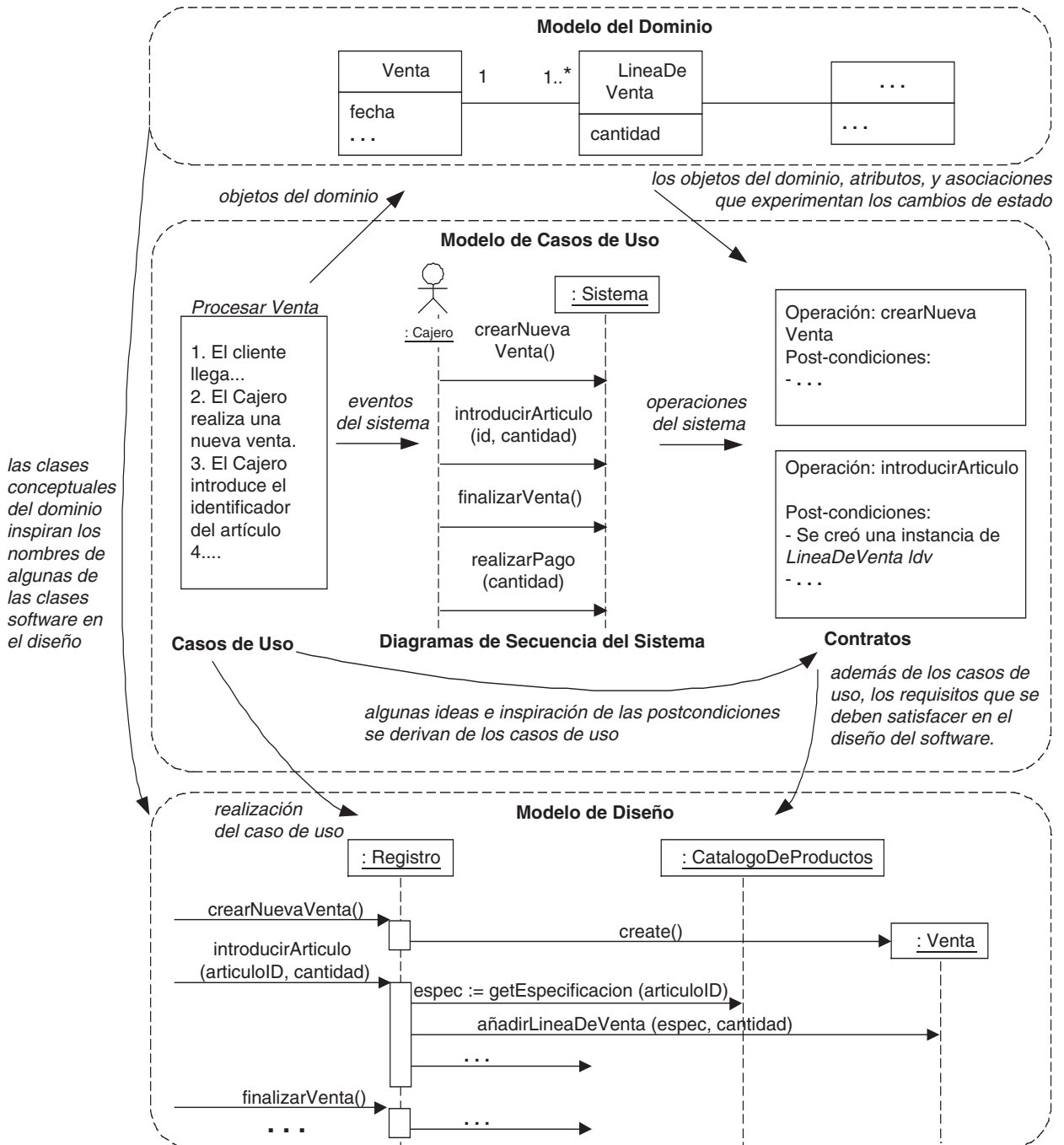
Figura 17.20. Muestra de la influencia entre los artefactos UP.
