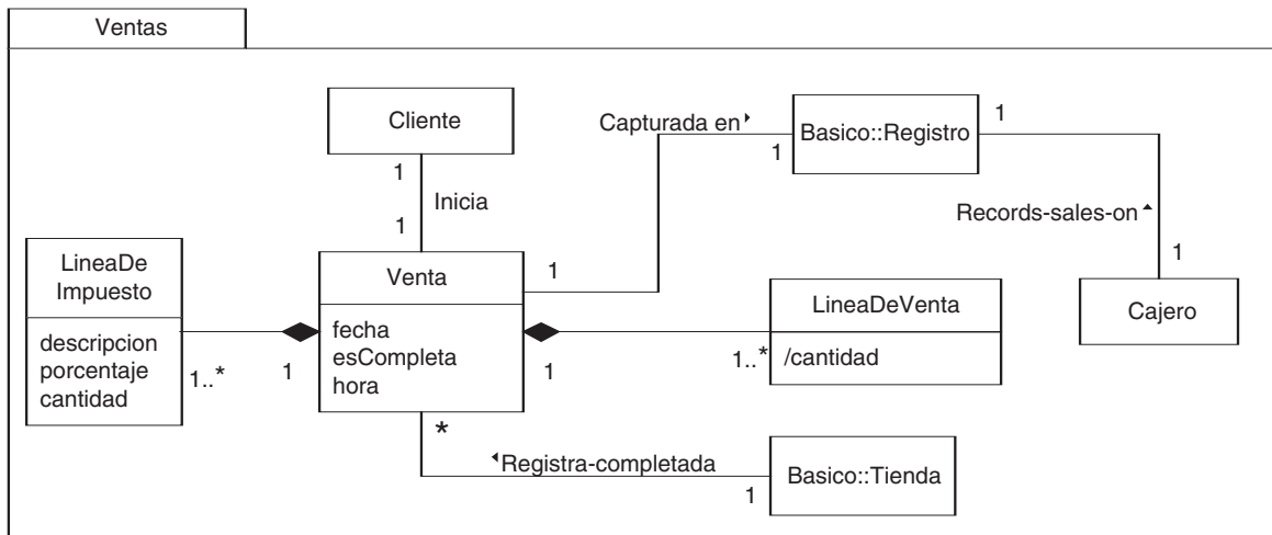
Figura 27.25. Paquete de ventas.
