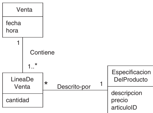
Figura 16.3. Asociaciones de Venta.
