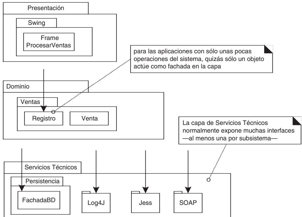
Figura 30.7. Número de interfaces que se muestran a las capas superiores.
