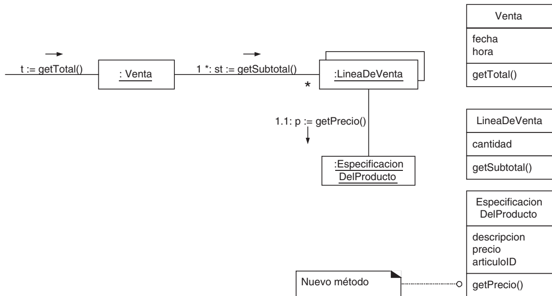
Figura 16.6. Cálculo del total de una Venta .
