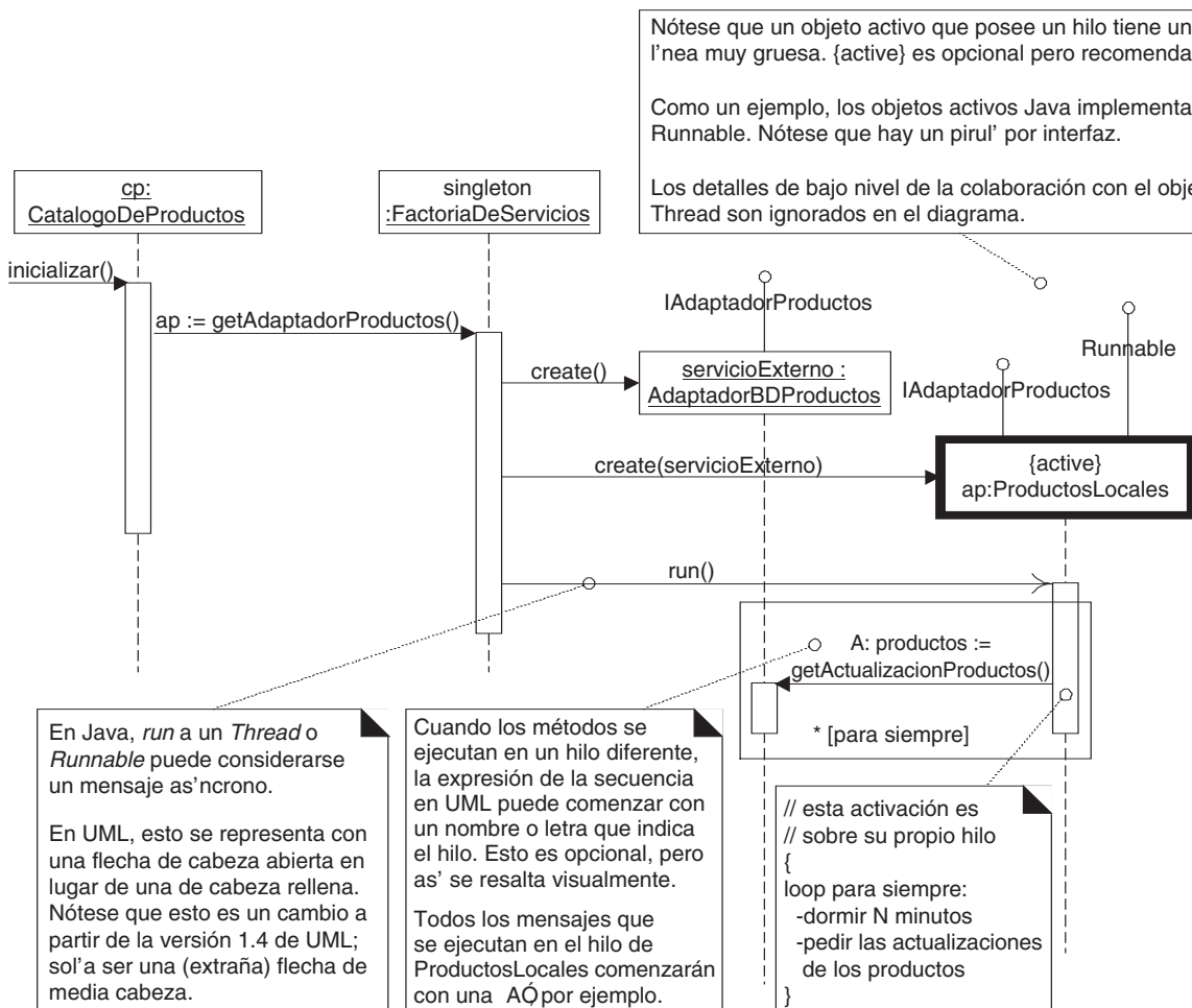
Figura 33.7. Hilos y mensajes asíncronos en UML.
