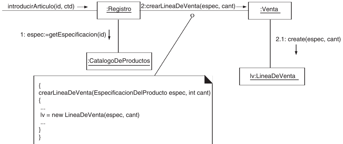
Figura 18.3. Visibilidad de parámetro.
