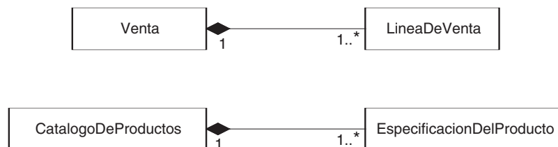
Figura 27.8. Agregación en la aplicación de punto de venta.
