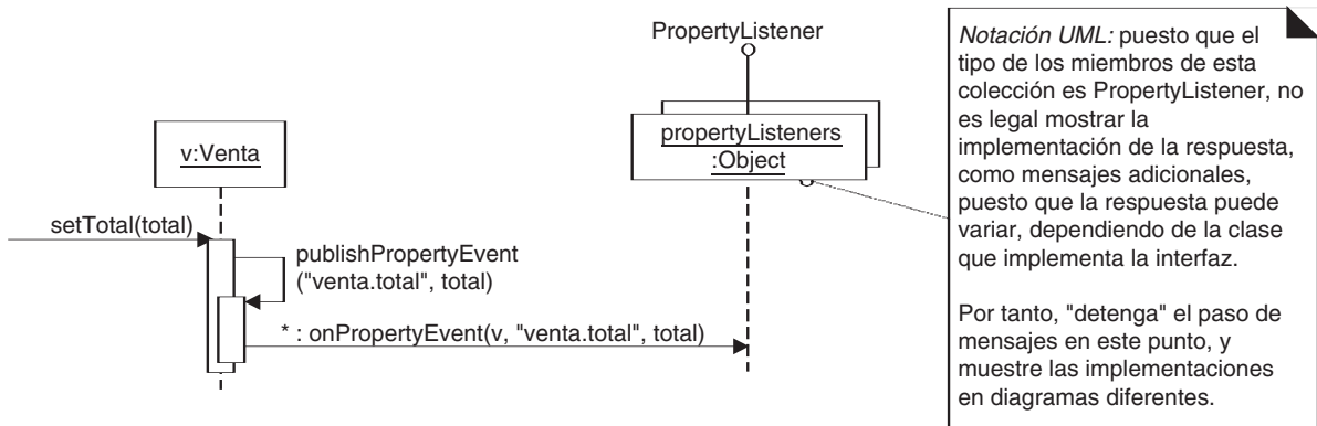
Figura 23.23. La Venta publica un evento sobre la propiedad a todos sus suscriptores.
