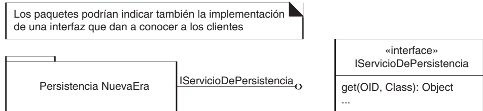
Figura 38.2. Interfaz de un paquete.
