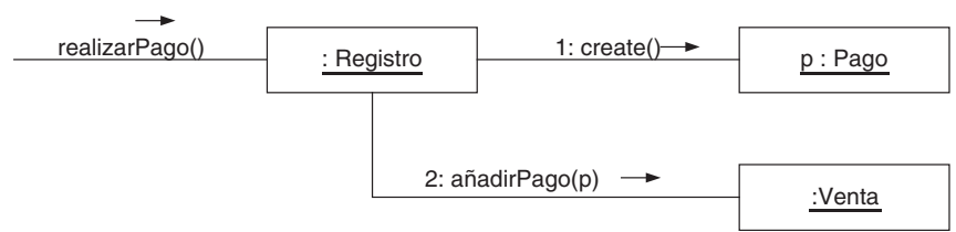
Figura 16.9. El Registro crea un Pago.
