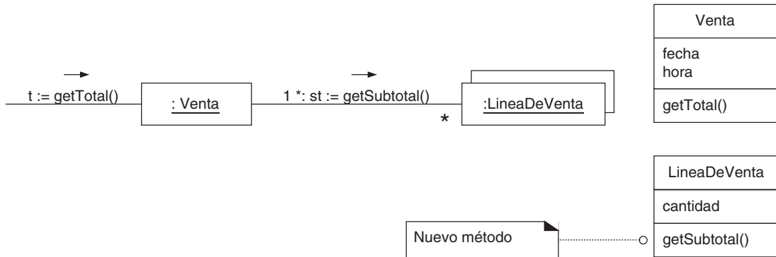
Figura 16.5. Cálculo del total de la Venta.
