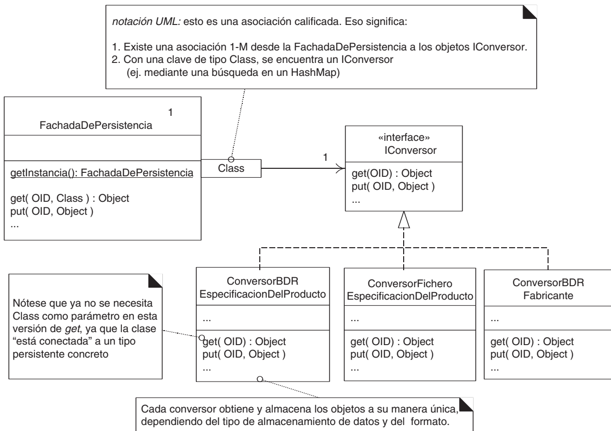
Figura 34.5. Conversores de bases de datos.
