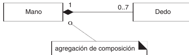
Figura 27.6. Agregación de composición.
