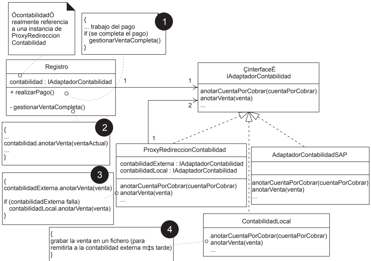
Figura 33.13. Uso en NuevaEra de un proxy de redirección.
