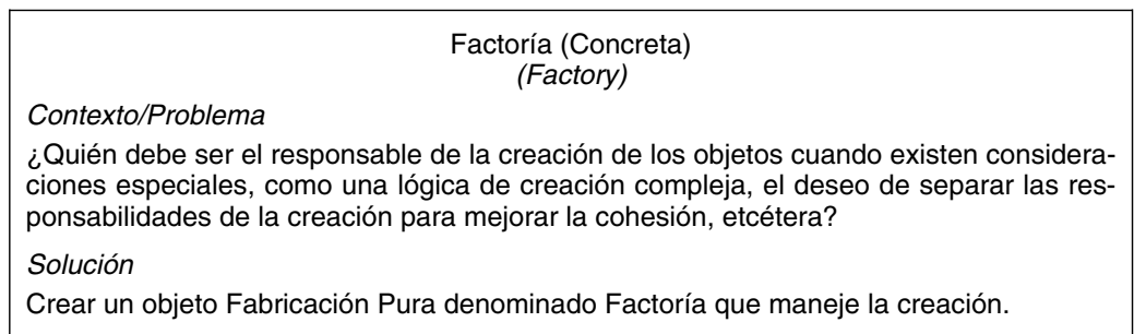
Figura 23.4. El patrón Factoría.
