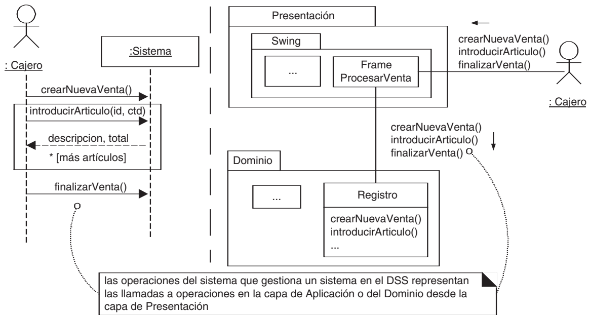
Figura 30.10. Operaciones del sistema en los DSS y en función de las capas.
