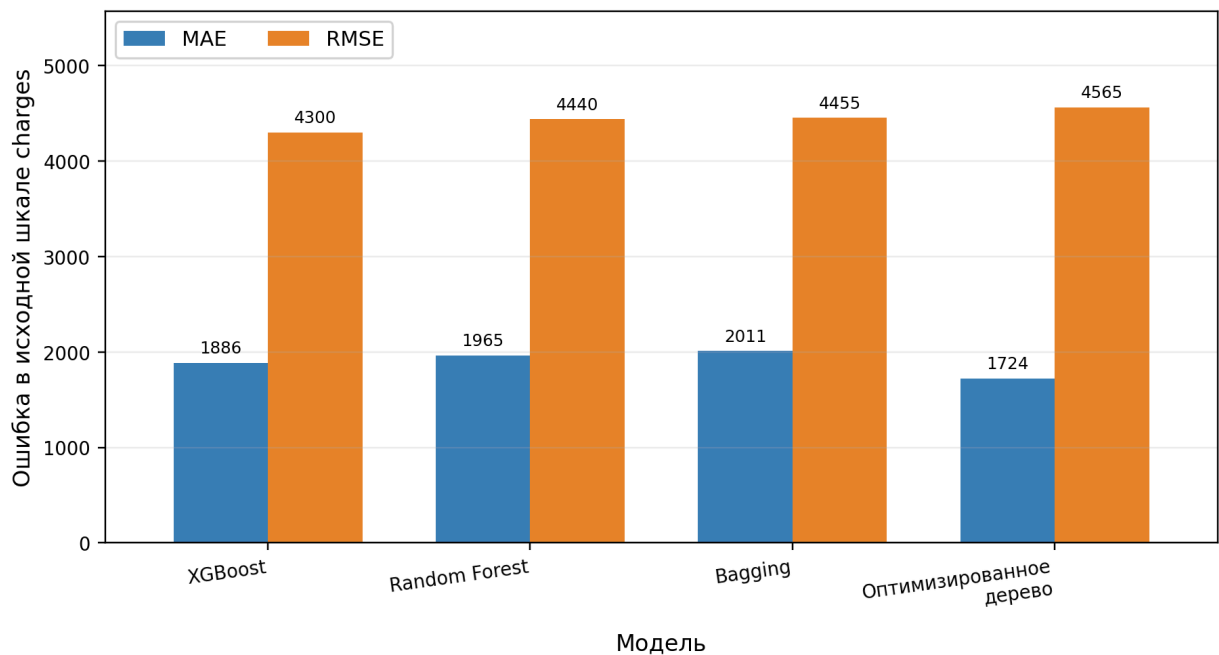
Рисунок 28 - Сравнение MAE и RMSE на тестовой выборке
