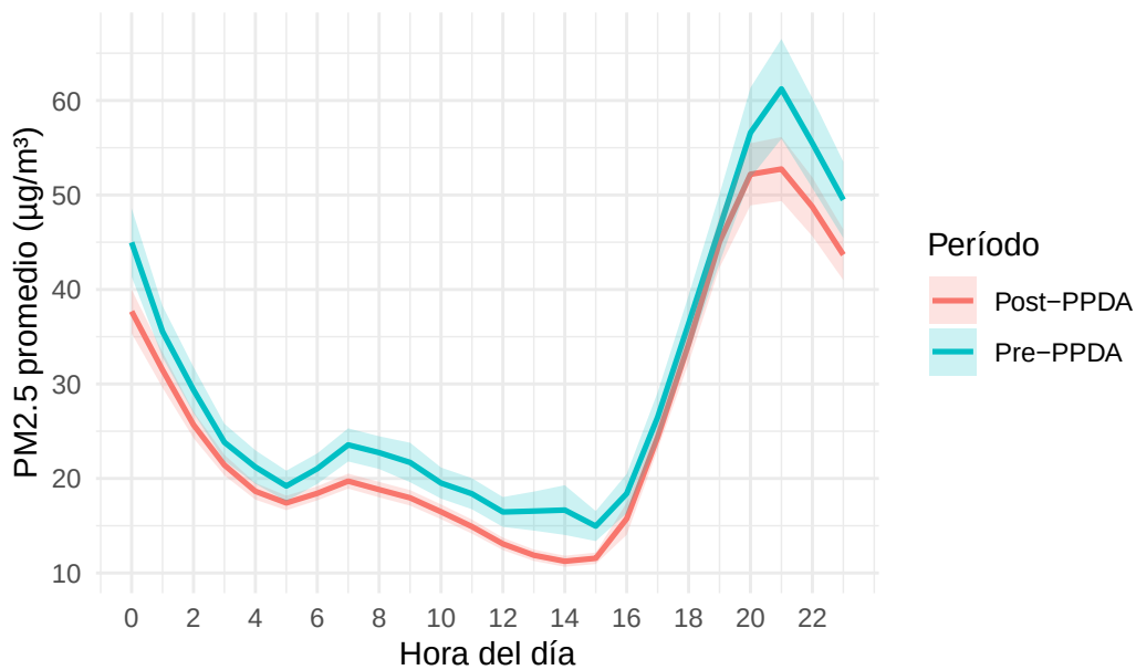
Perfil diario de PM 2.5 – estación TALI
