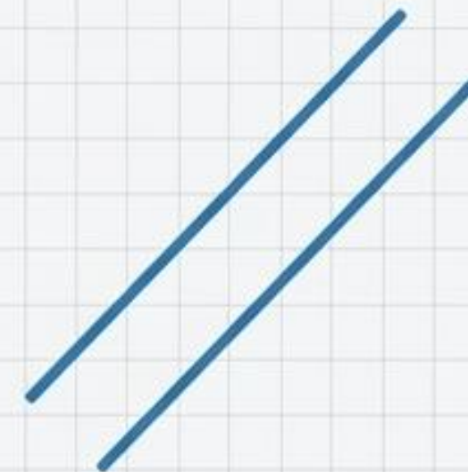
успоредни прави
