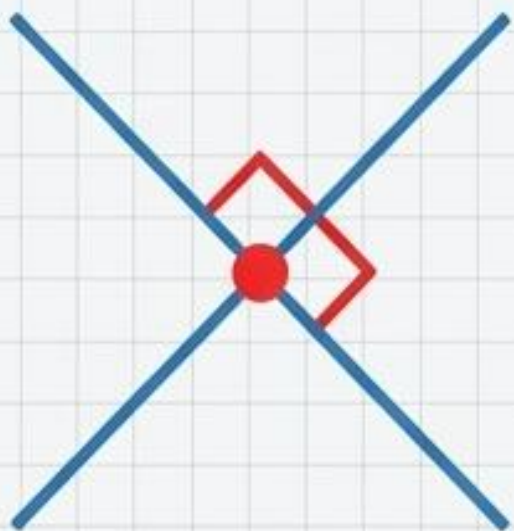
перпендикулярни приви
