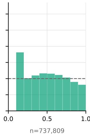
EMOS local
