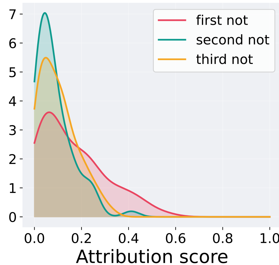
SHAP
