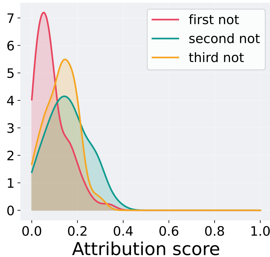
LIME
