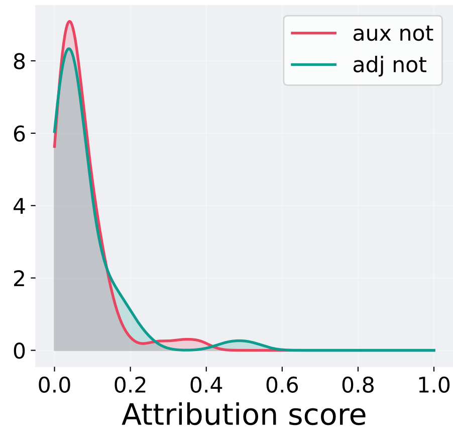
IG
