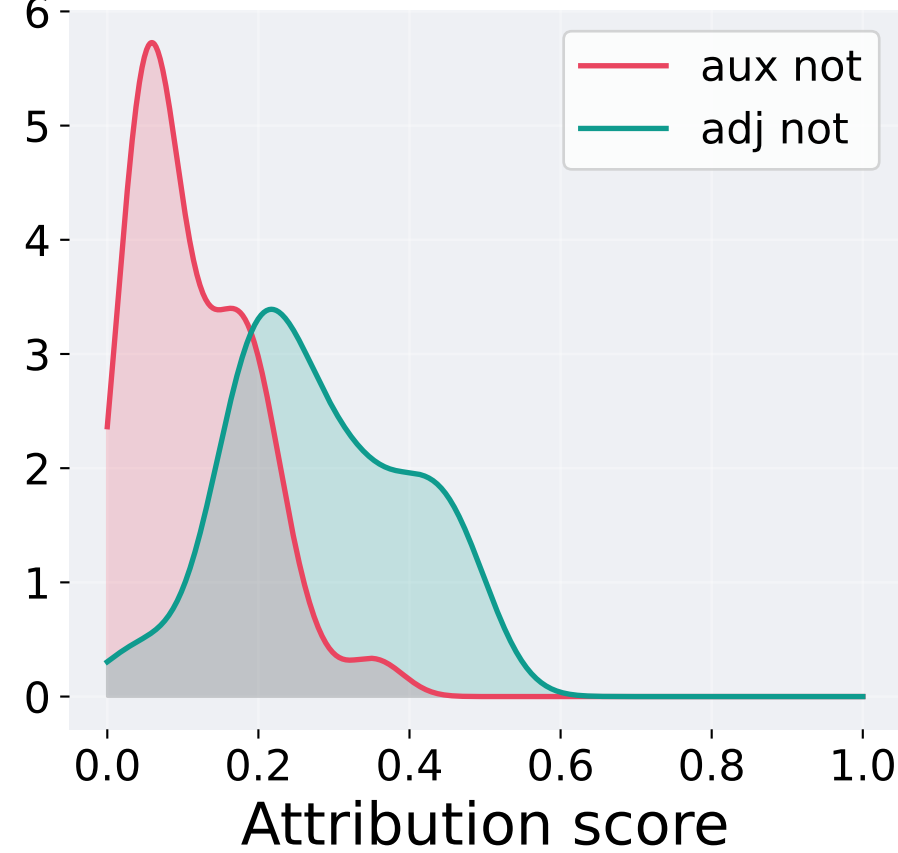
LIME
