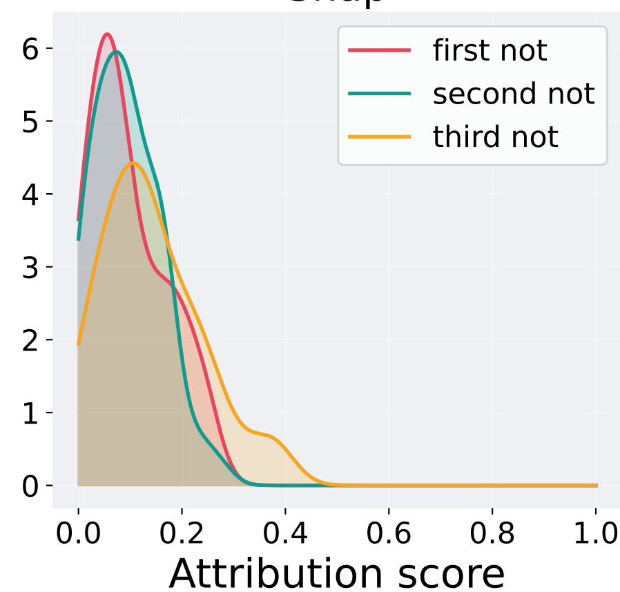
Shap
