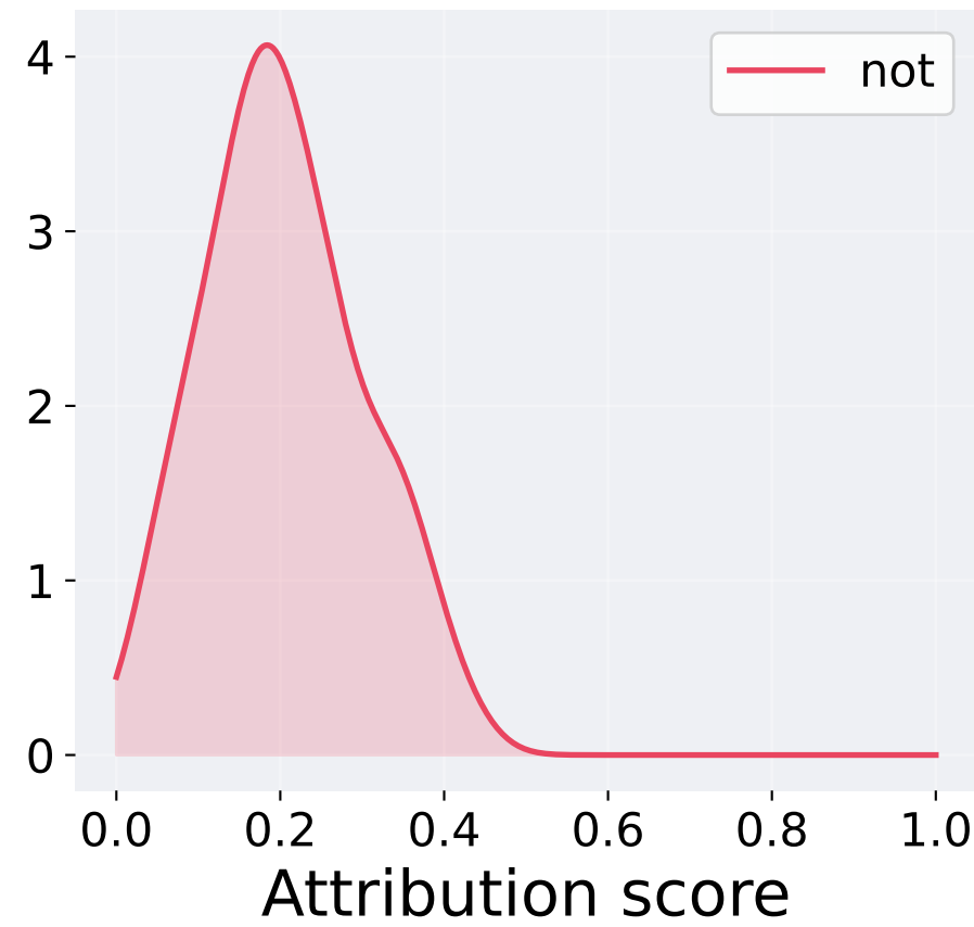
LIME
