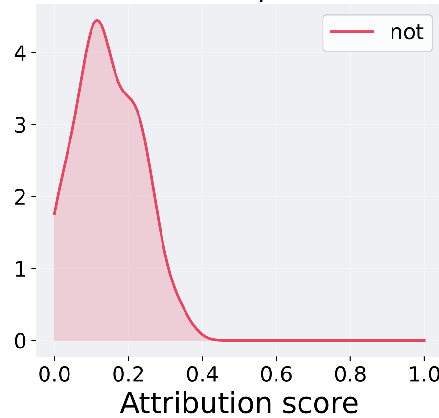
Shap
