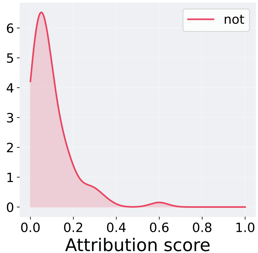
IG
