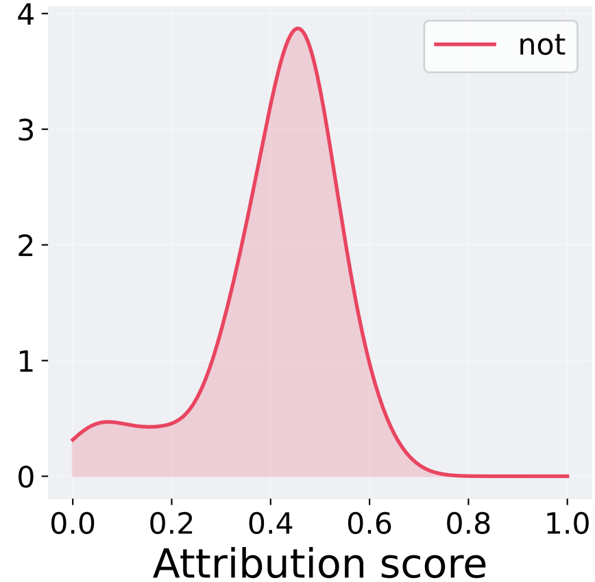
LIME
