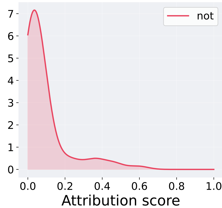
SHAP
