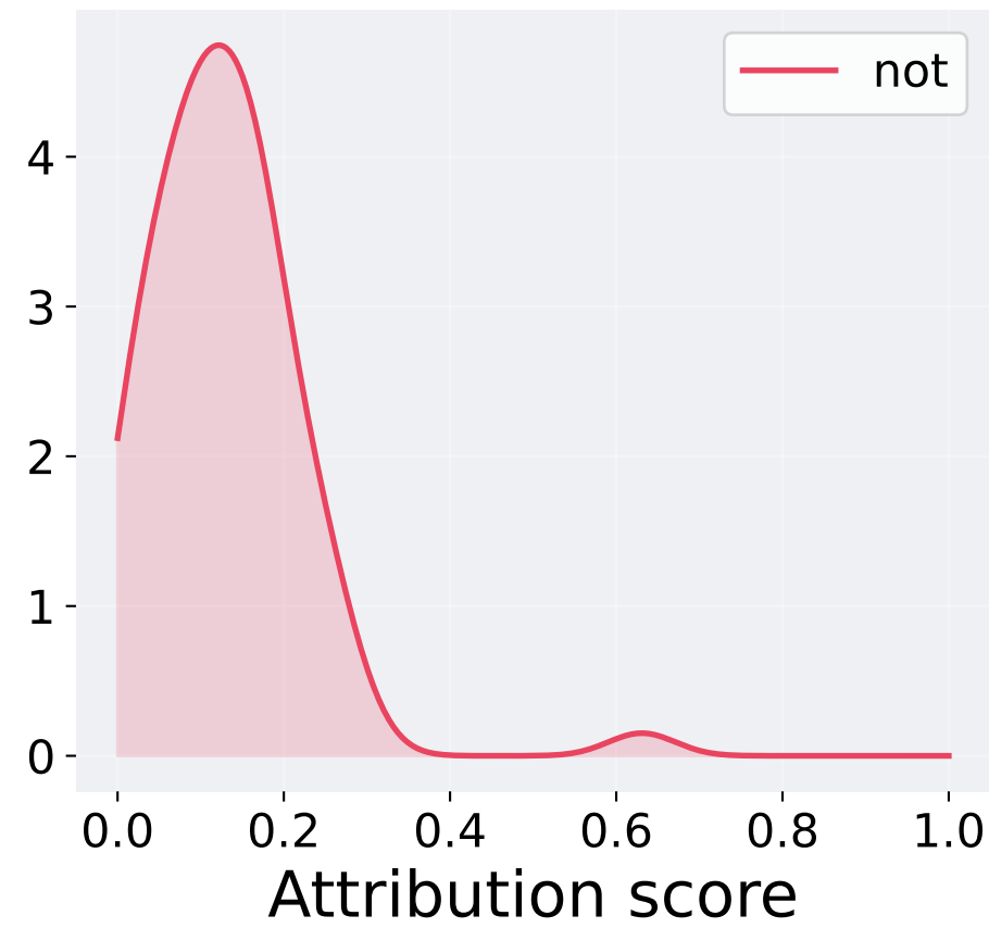
LIME
