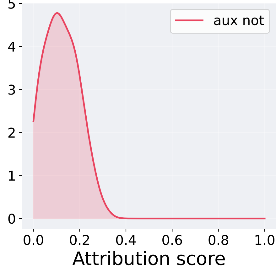
LIME
