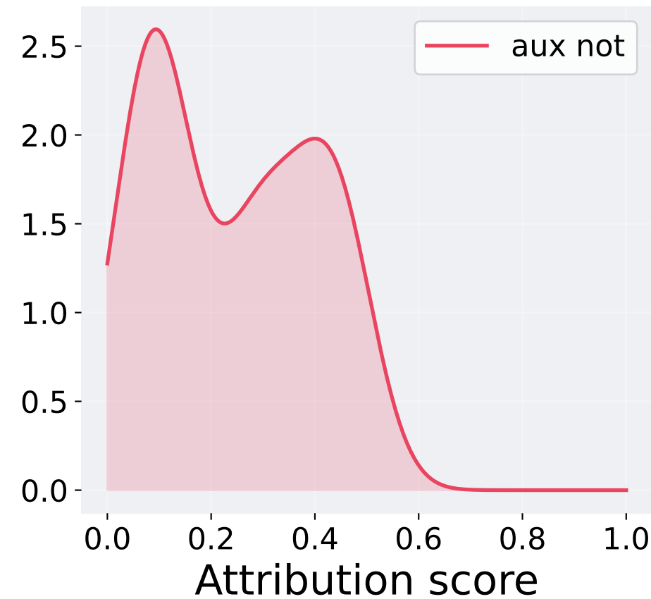
SHAP
