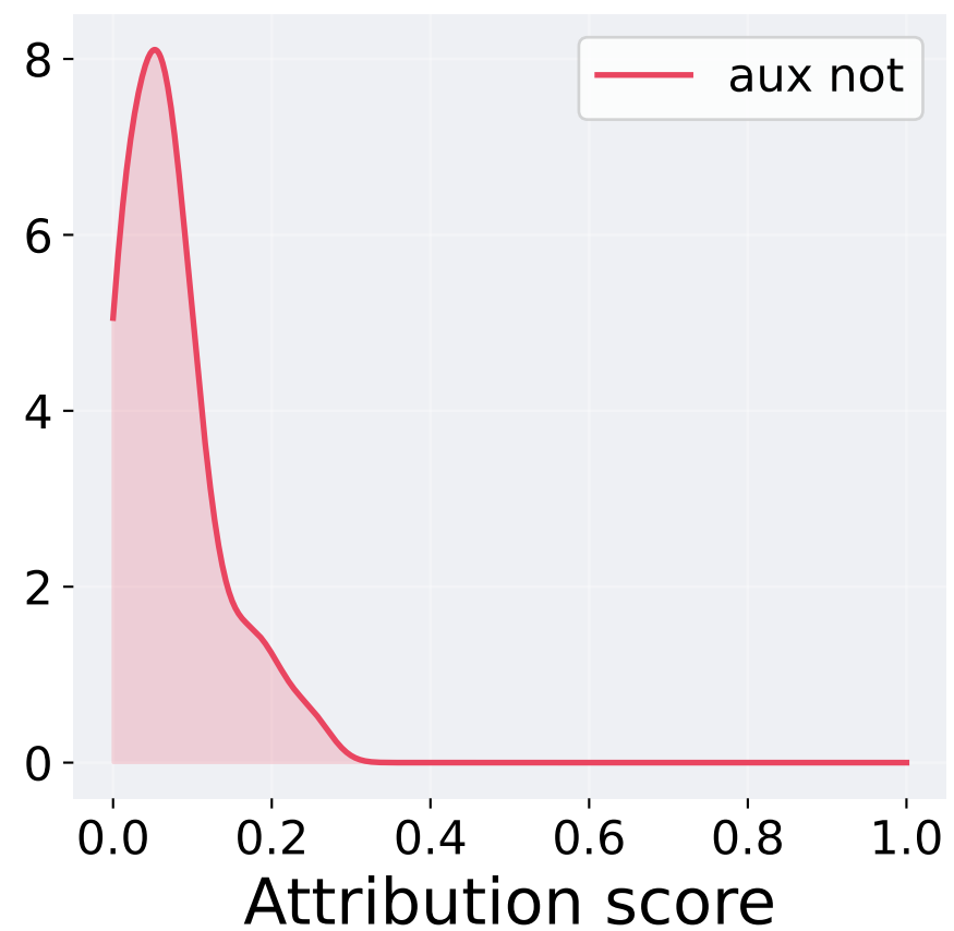
IG
