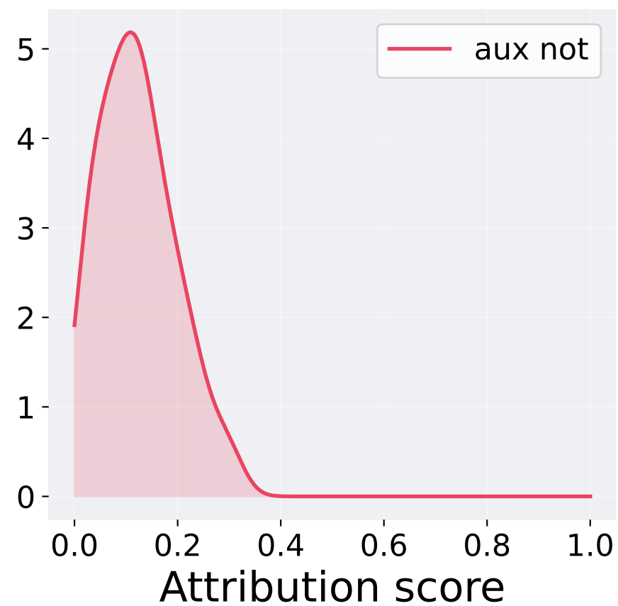
LIME
