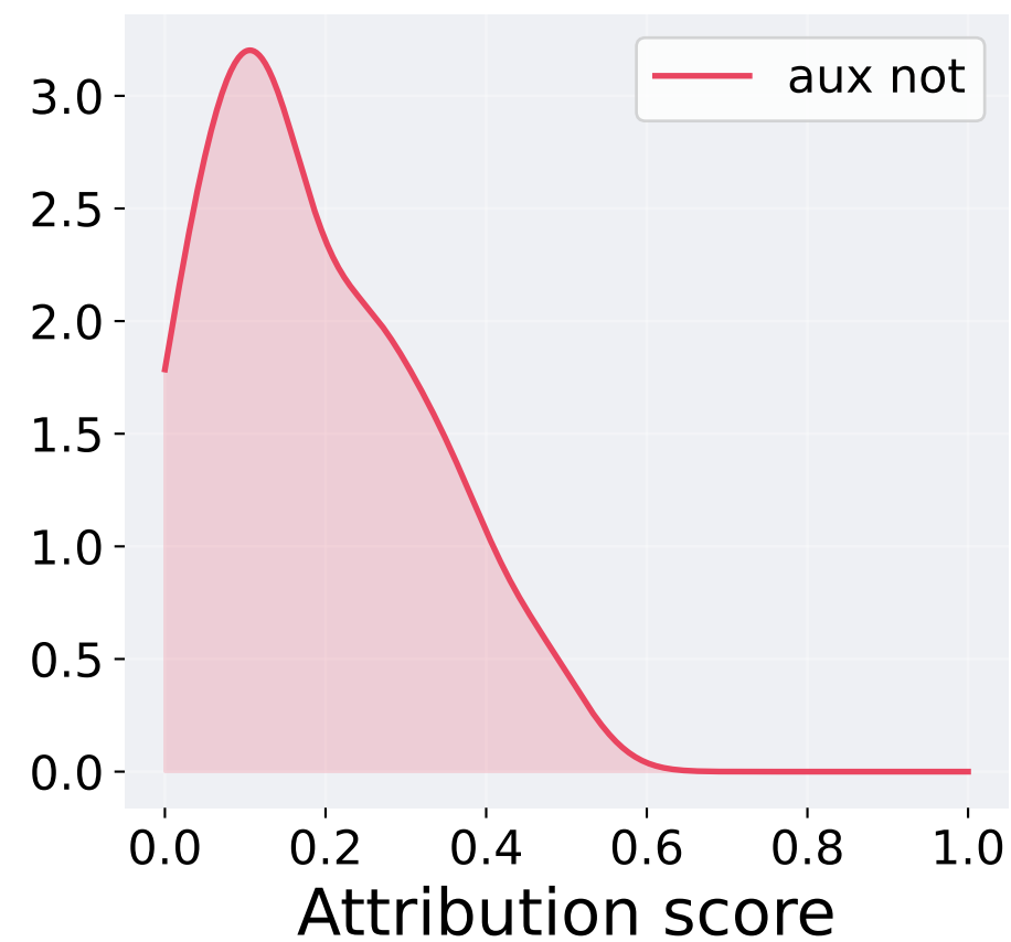
SHAP
