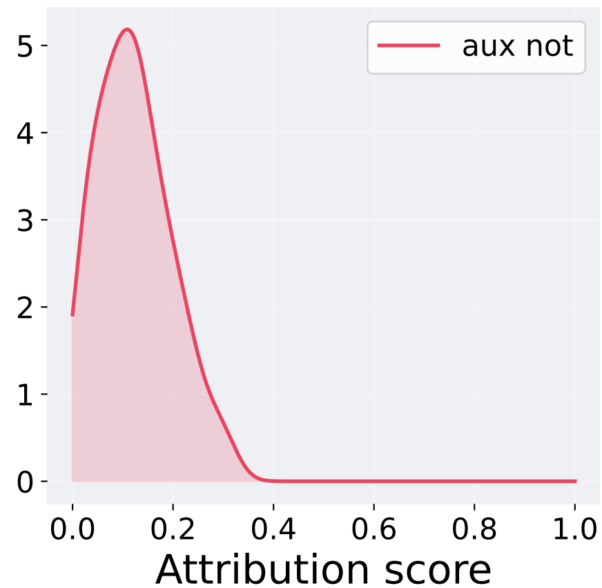
LIME
