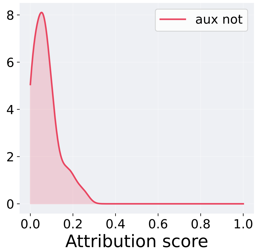
IG
