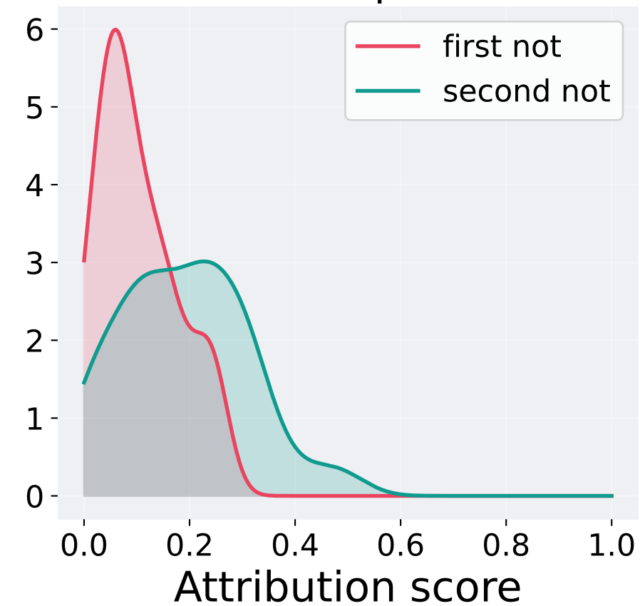
Shap
