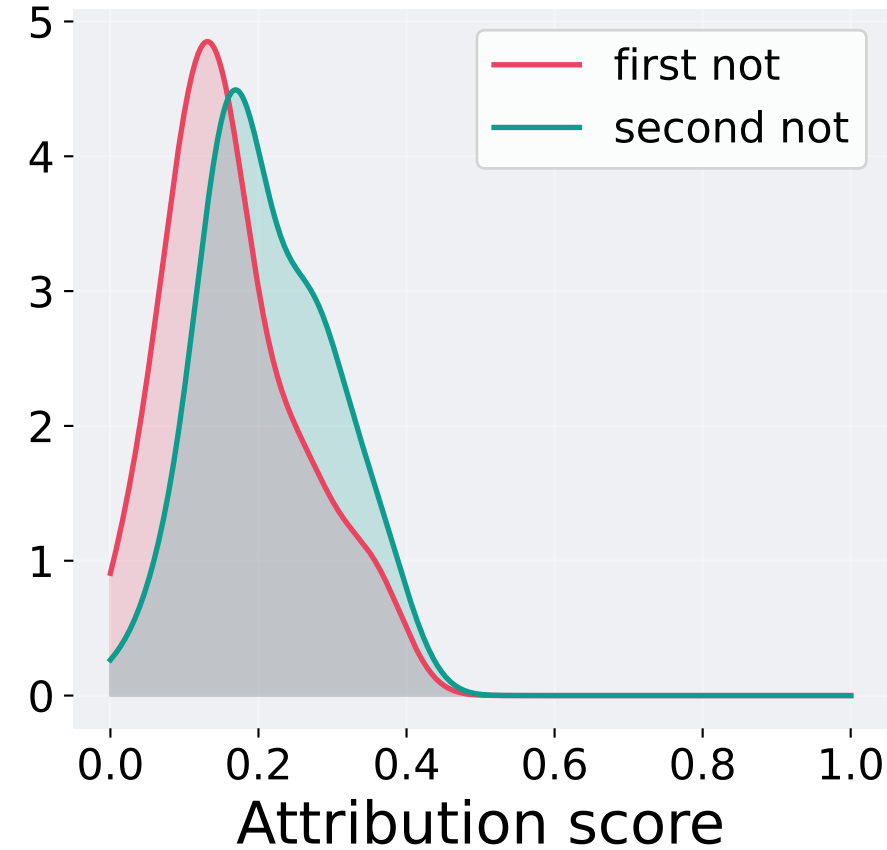
LIME
