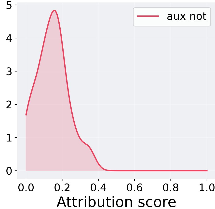
LIME
