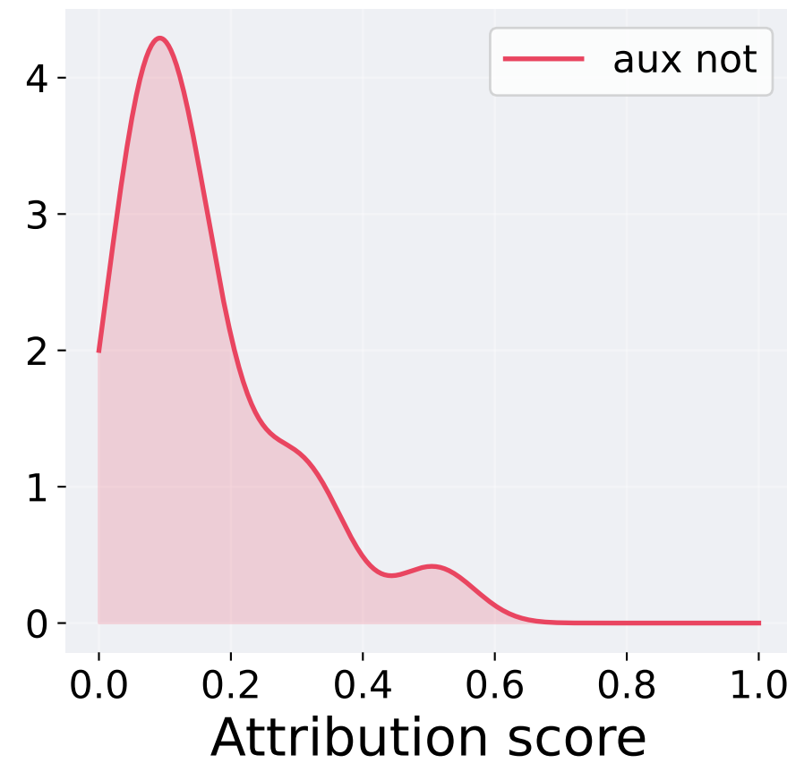
SHAP
