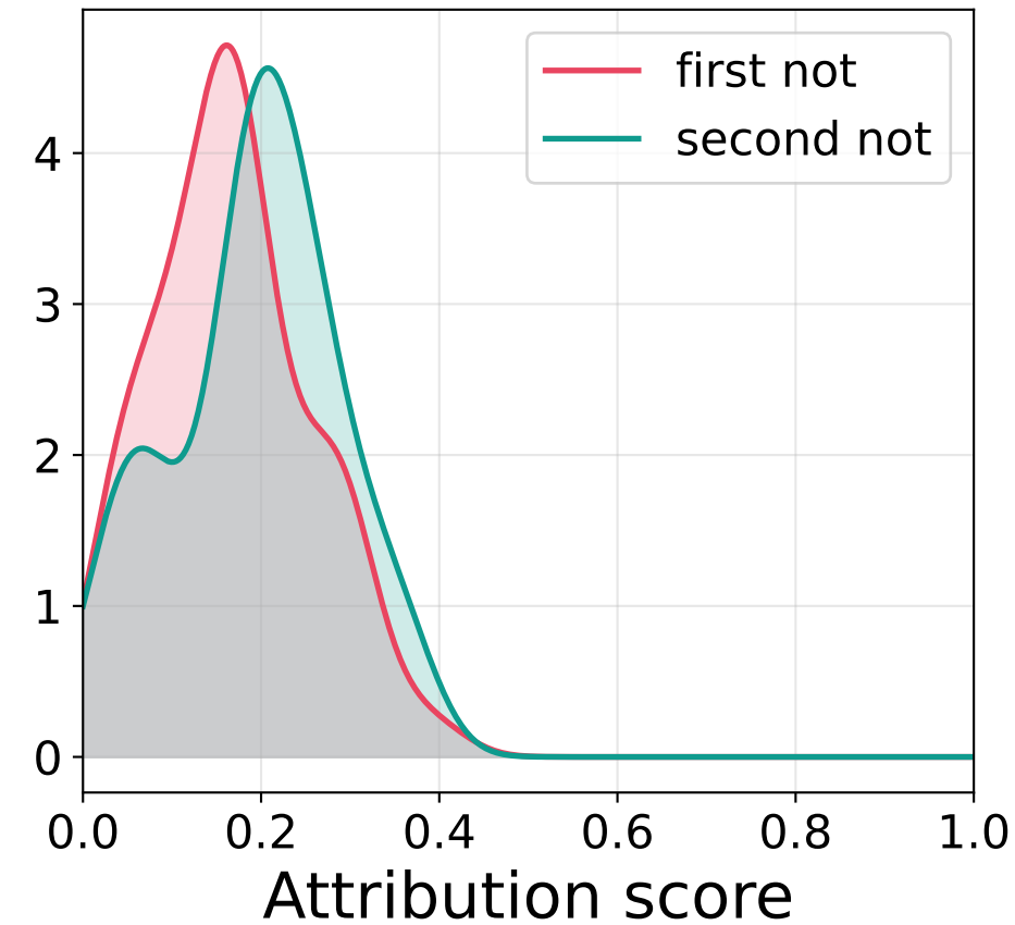
LIME
