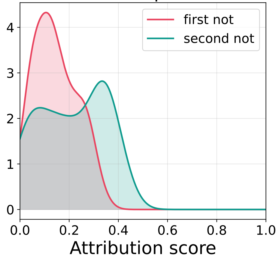
Shap
