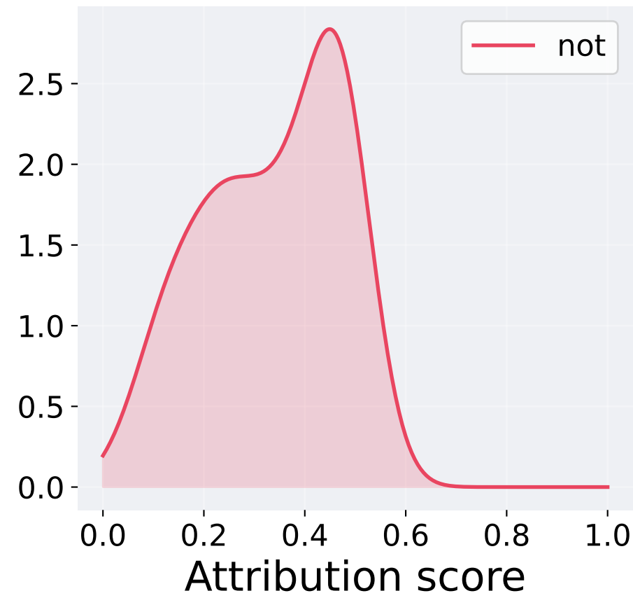
LIME
