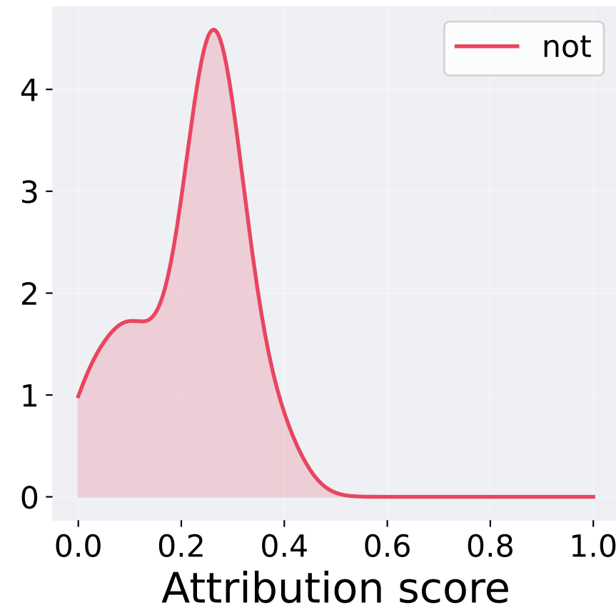
SHAP
