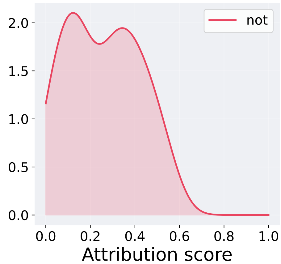
IG
