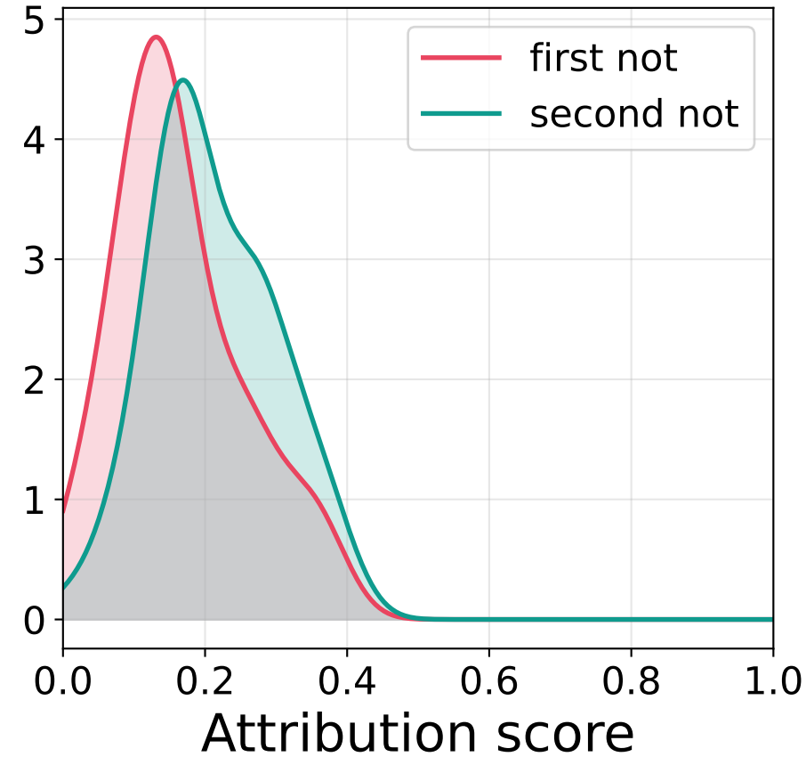
LIME
