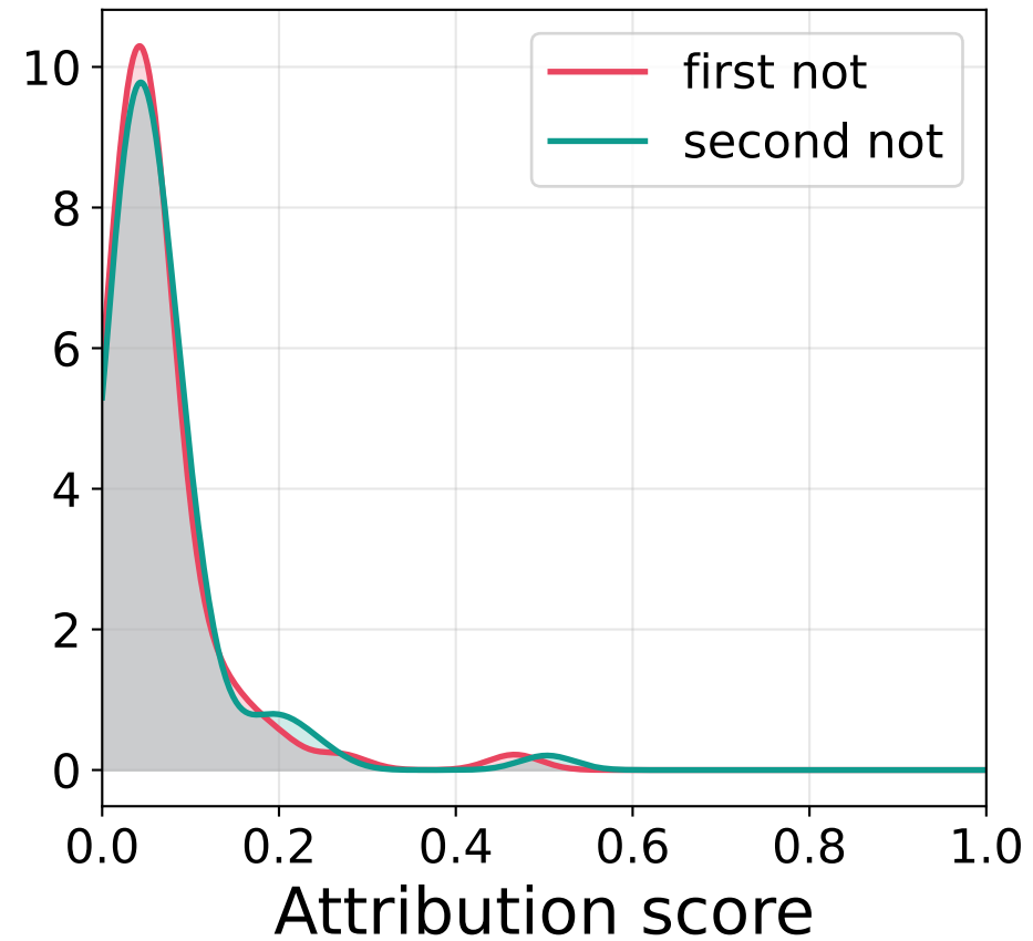
IG
