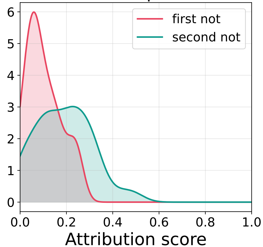
Shap
