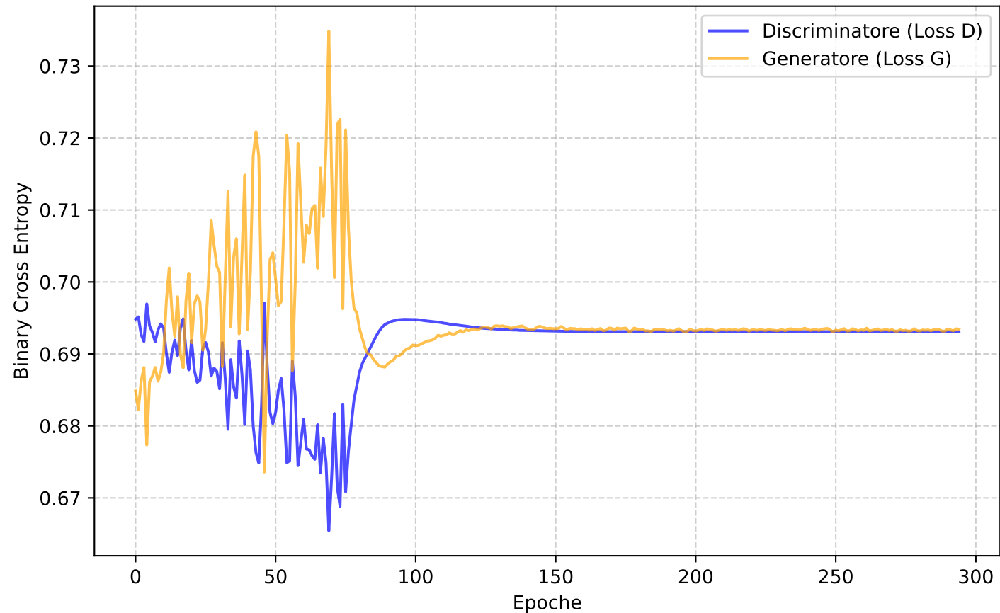
Dinamica Avversaria (GAN Losses)
