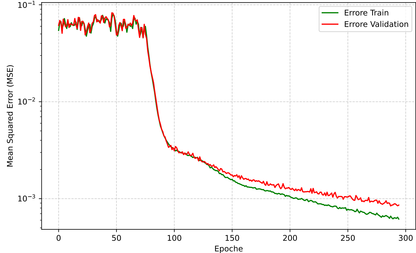
Ricostruzione Matrice Densità (Train e Validation)
