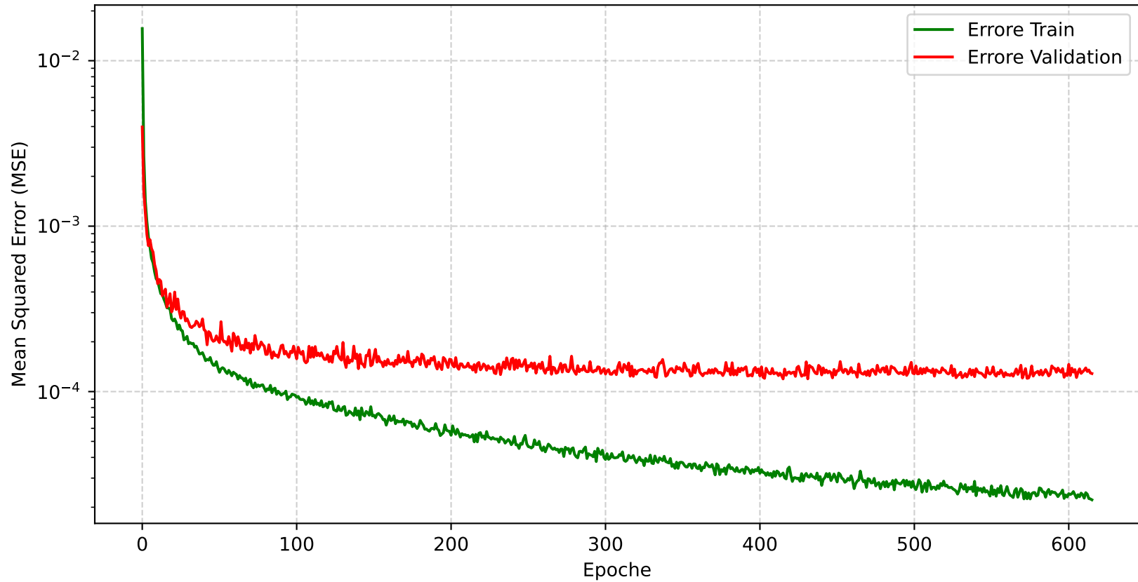
Errori di Train e Validation
