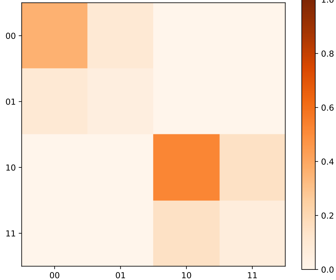
QST-CGAN (Parte Reale)
