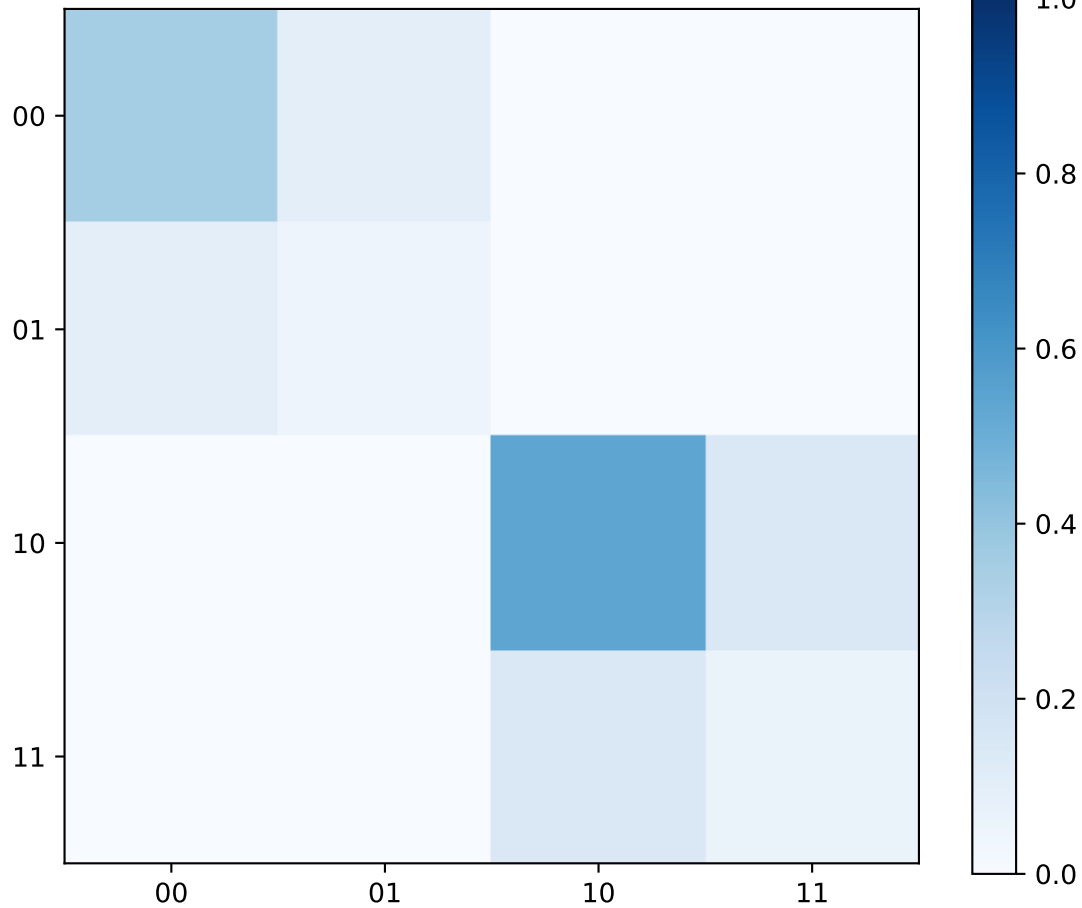
True Matrix (Parte Reale)
