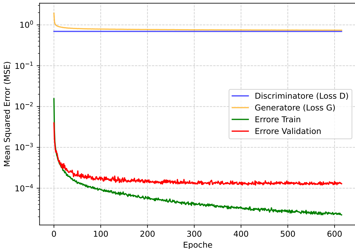
Errori di Train e Validation
