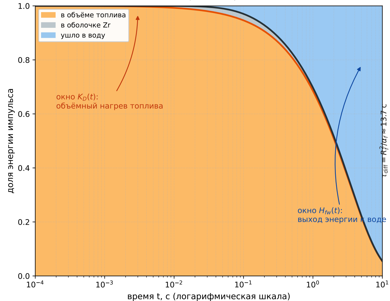
(б) Разделение энергии импульса по объёмам
