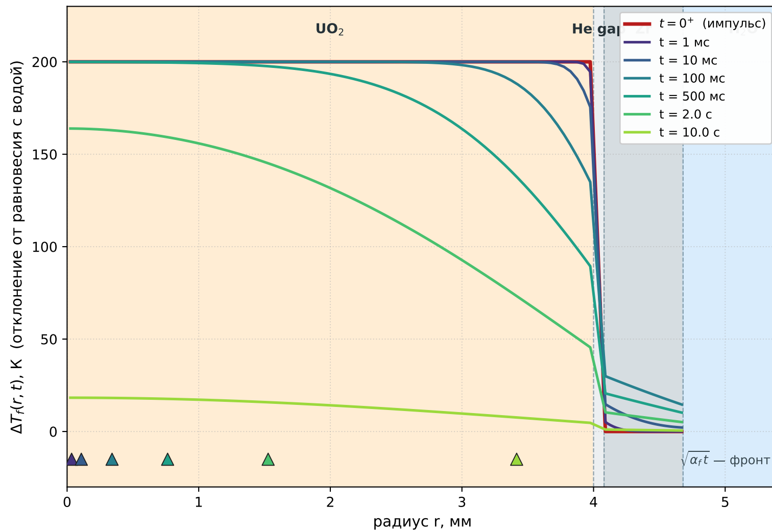
(а) Радиальная релаксация теплового следа \Delta T_f(r, t)
